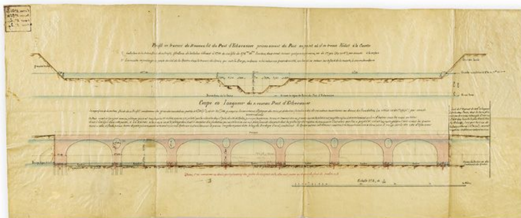
Profil en travers du Nouveau lit du Pont d'Echavannes. Coupe en longueur du nouveau Pont d'Echavannes. 71, Chalon-sur-Saône route départementale 19
