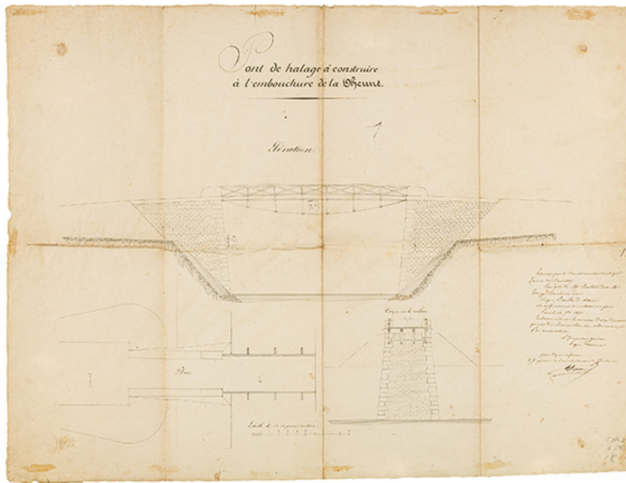
Pont de halage à construire à l'embouchure de la Dheune. Plan, coupe et élévation. Dessin, 30 août 1837. 71, Bragny-sur-Saône, lieudit : PK 165,3
