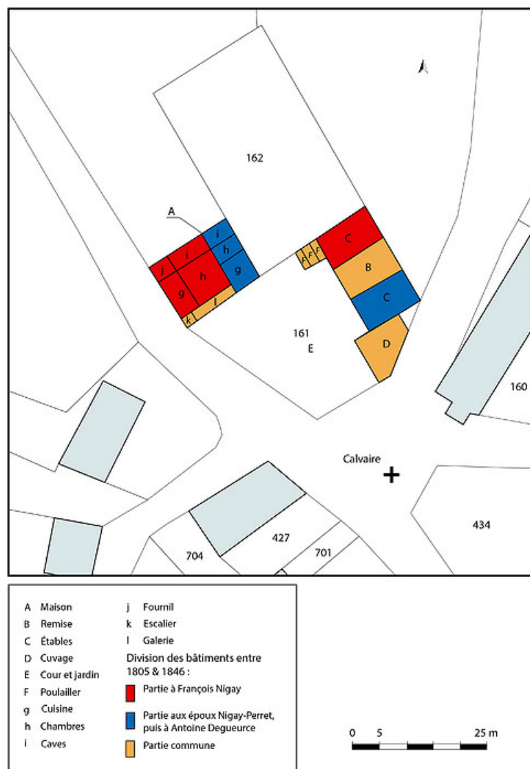
Plan de masse et de situation, présentant l'évolution des bâtiments. Extrait du plan cadastral, 2020, section B, échelle 1/2500 71, Vauban, lieudit : la Place
