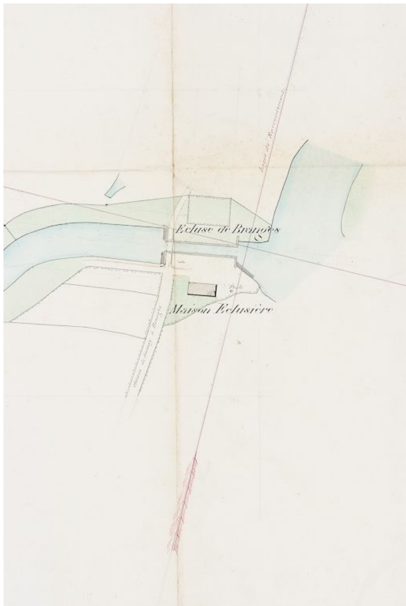
La Seille : profils de Louhans à La Truchère. Détail du site d'écluse de Branges. (Archives VNF-direction territoriale Centre-Bourgogne ; subdivision de Montceau-les-Mines)
