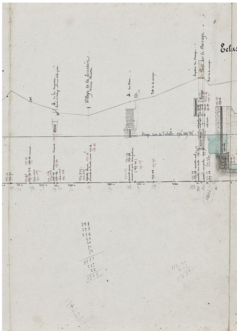
"Nivellement de la Seille, profils", par l'ingénieur Fournier, vers 1850. Croquis non datés des ponceaux et aqueducs du chemin de halage. Extrait : Aqueducs et ponceaux, km 1 et 2. (Archives VNF-direction territoriale Centre-Bourgogne ; subdivision de Montceau-les-Mines)
