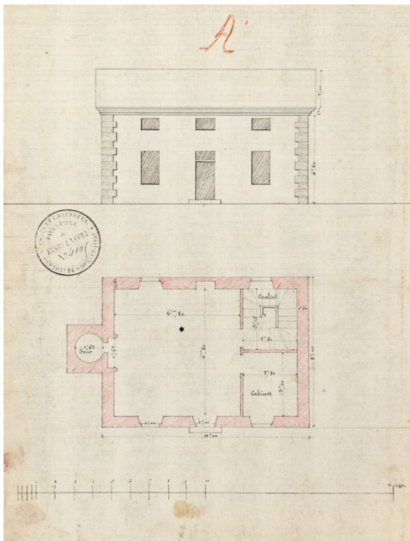
Elévation et plan d'une maison éclésièr de la Seille. Ce plan non daté, non signé a permis de construire la maison de Branges. (Archives VNF-direction territoriale Centre-Bourgogne ; subdivision de Montceau-les-Mines)
