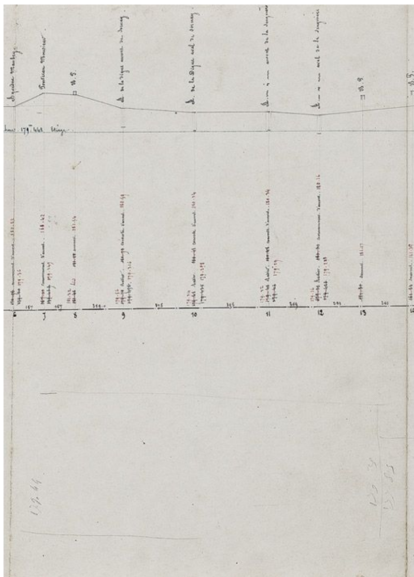
"Nivellement de la Seille, profils", par l'ingénieur Fournier, vers 1850. Croquis non datés des ponceaux et aqueducs du chemin de halage. Extrait : Partie sur la commune de Sornay. (Archives VNF-direction territoriale Centre-Bourgogne ; subdivision de Montceau-les-Mines)
