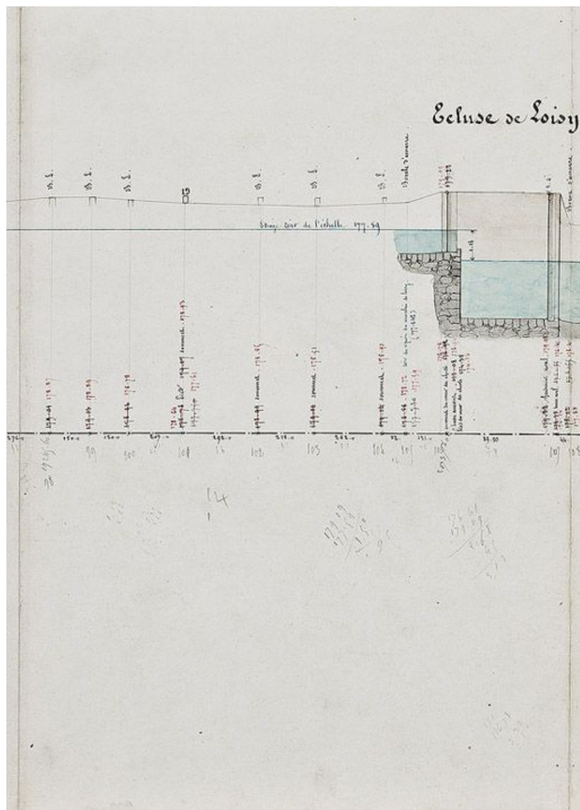
"Nivellement de la Seille, profils", par l'ingénieur Fournier, vers 1850. Croquis non datés des ponceaux et aqueducs du chemin de halage. Extrait : km 19 et écluse de Loisy. (Archives VNF-direction territoriale Centre-Bourgogne ; subdivision de Montceau-les-Mines)
