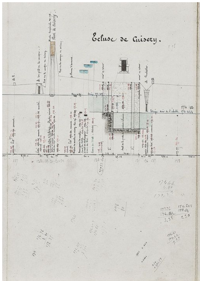
"Nivellement de la Seille, profils", par l'ingénieur Fournier, vers 1850. Extrait : Ecluse de Cuisery (Archives VNF-direction territoriale Centre-Bourgogne ; subdivision de Montceau-les-Mines)
