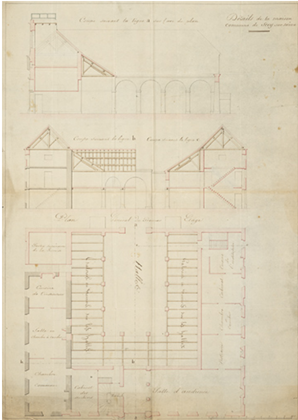
Duret. Détails de la maison commune de Sceaux-sur-Saône. Coupe. Plan général du premier étage. [1831]. 70, Sceaux-sur-Saône-et-Saint-Albin, 24-26-30-32 rue Armand Paulmard
