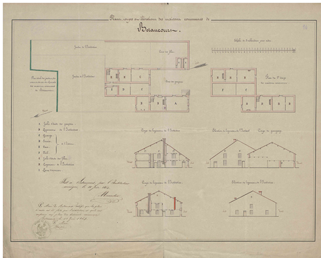
Plans, coupes et élévations des maisons communes de Bataucourt. Fait par l'instituteur le 10 juin 1864. 70, Bataucourt
