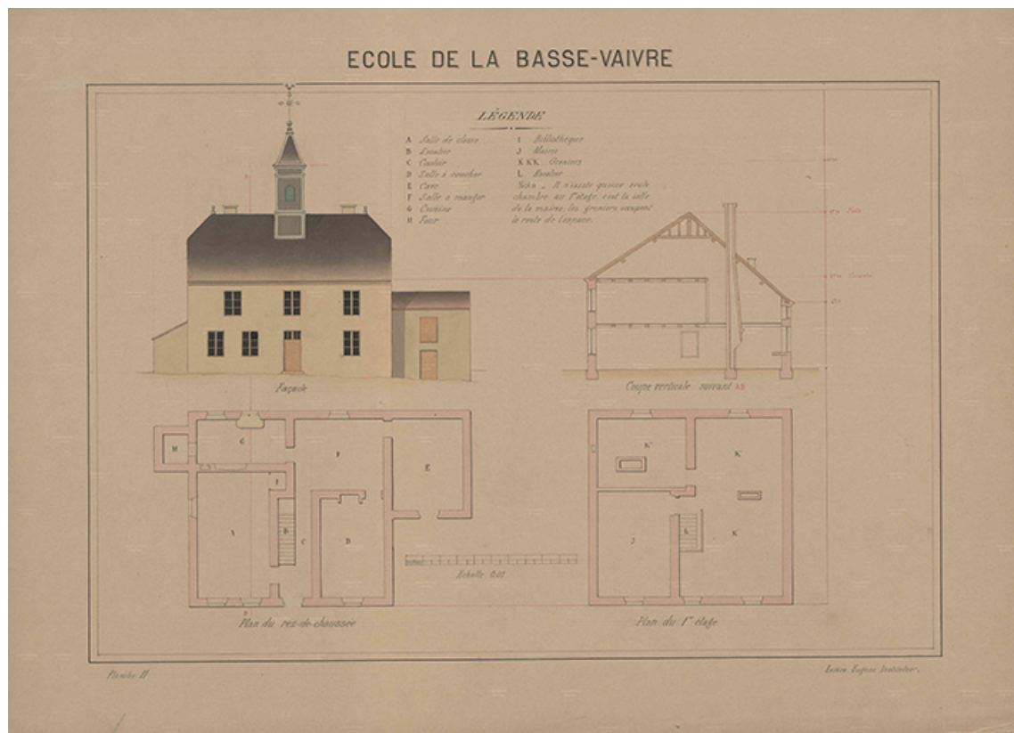
École de la Basse Vaivre. Dessin et légende. 1888.
