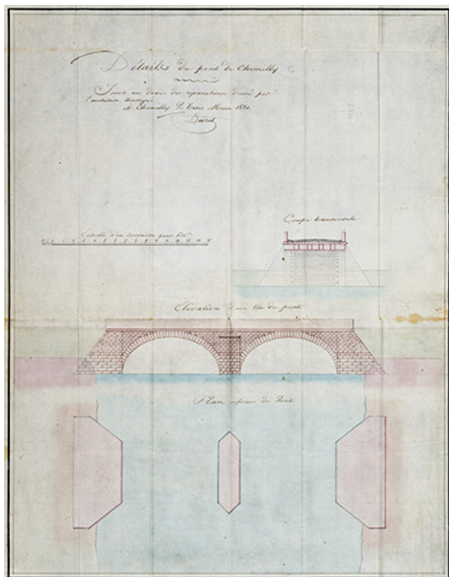
Plans du pont à établir sur le Durgeon, 1831 70, Chemilly
