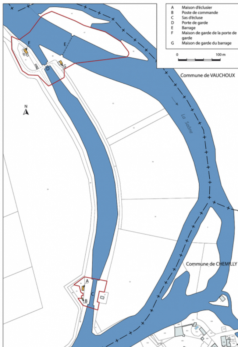
Plan masse et de situation. Détail sud du bief incluant porte de garde et site d'écluse aval. 70, Ferrières-lès-Scey
