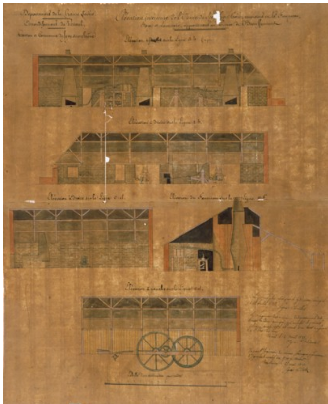
Elévation intérieure de l'usine de Scey-sur-Saône consistant en haut fourneau, forges et laminoir [...].
