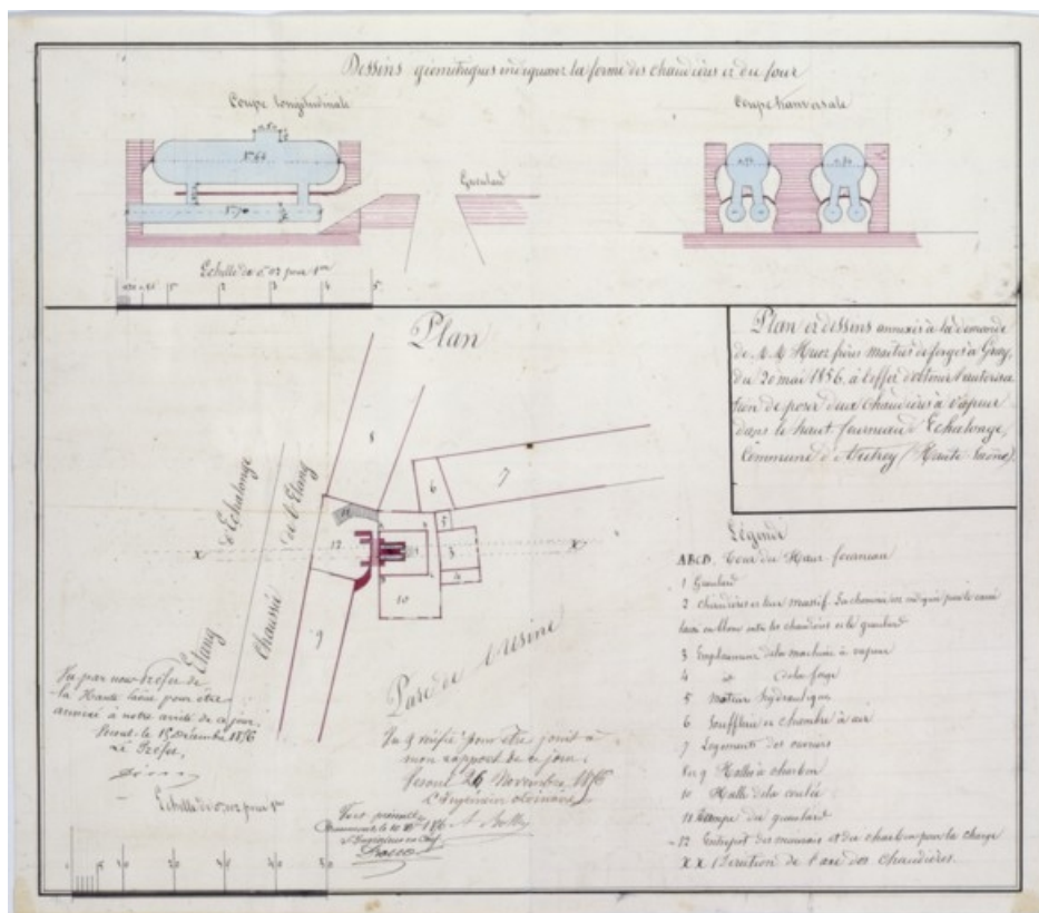
Plans et dessins annexés à la demande de MM. Huot frères [...] à l'effet d'obtenir l'autorisation de poser deux chaudières à vapeur [...].
