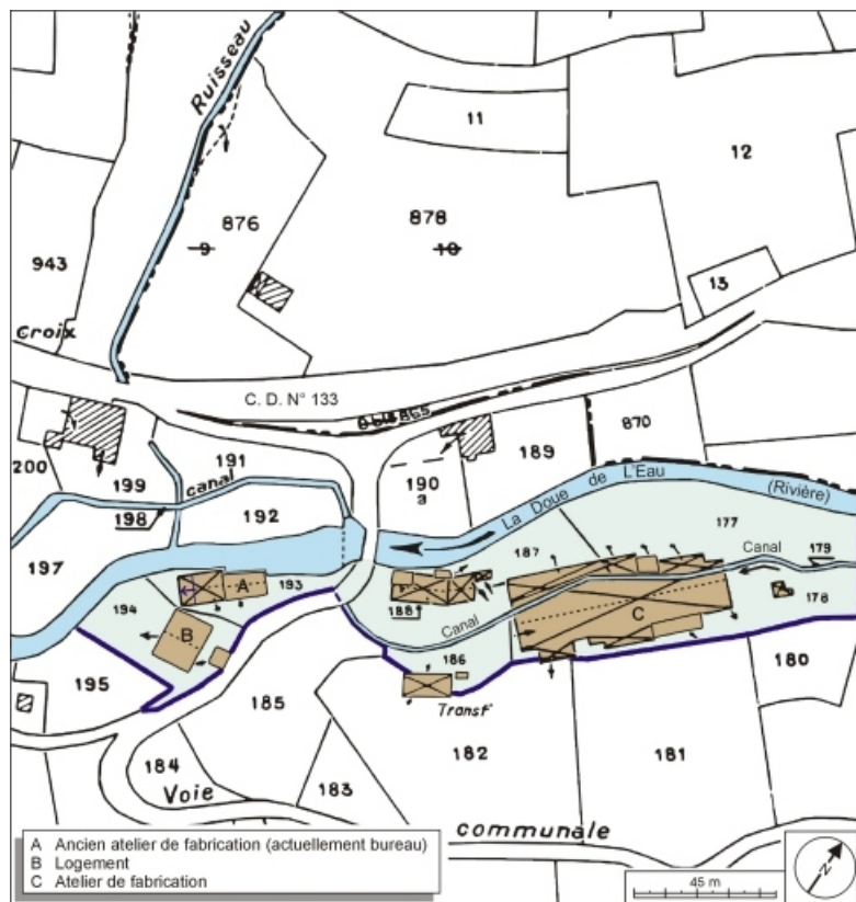
Plan-masse et de situation. Extrait du plan cadastral numérisé, 2005, section B, 1:2000 agrandi à 1:1500. 70, Miellin, lieudit : la Forge
