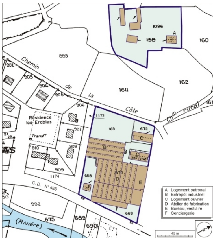
Plan-masse et de situation. Extrait du plan cadastral numérisé, 2005, section H, 1:2000 agrandi à 1:1500. 70, Mélisey, 54 à 58 route de Lure
