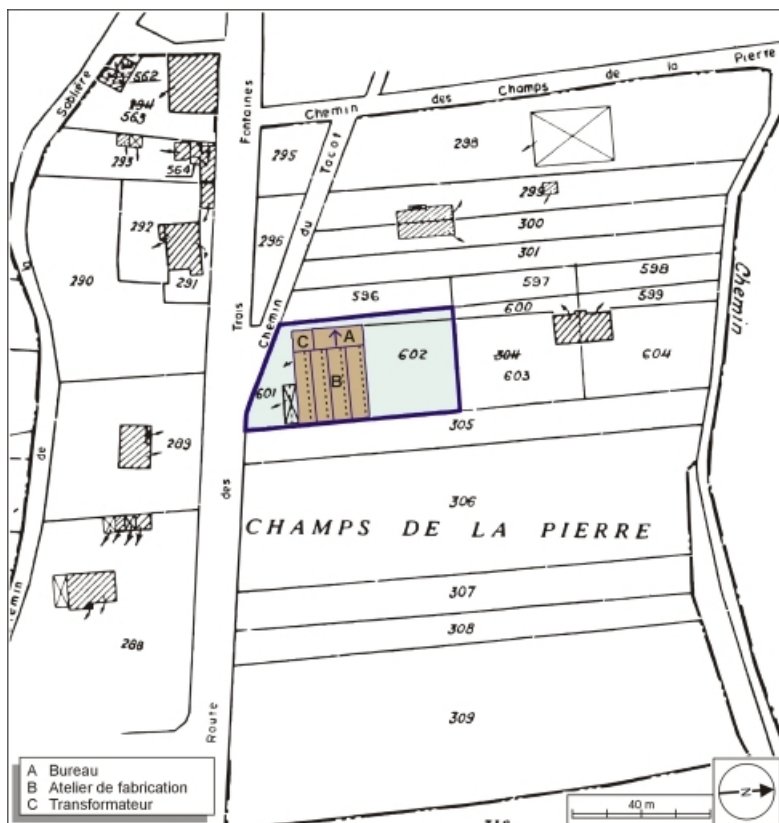
Plan-masse et de situation. Extrait du plan cadastral numérisé, 2005, section B, 1:1250. 70, Amage R.D. 6
