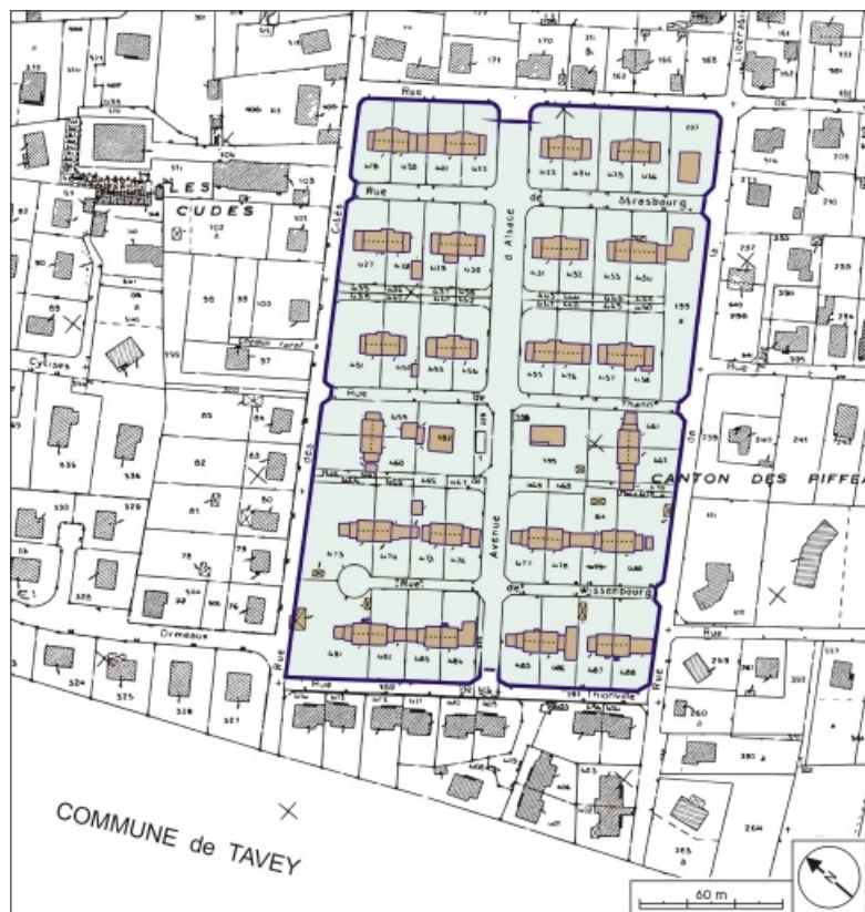
Plan-masse et de situation. Extrait du plan cadastral numérisé, 2005, section AS, 1:1000 réduit à 1:2000. 70, Héricourt rue des Cités Dollfus
