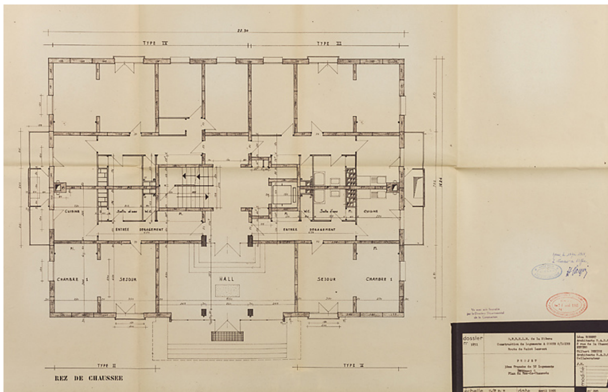
Bâtiment A à K : troisième tranche de 52 logements, bâtiment G, plan du rez-de-chaussée ; L. Robert, G. Denise, avril 1965. (Archives municipales Cosne-Cours-sur-Loire, 200 W 20 - PC 821)
