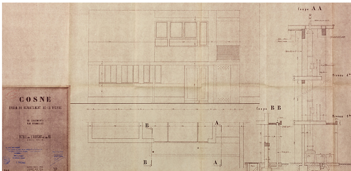
Opération de 32 logements, plan et élévations de détail de l'auvent et du vide-ordure, L. Robert et M. Guillaume, avril 1955. (Archives municipales Cosne-Cours-sur-Loire, 200 W 16 - PC 722)
