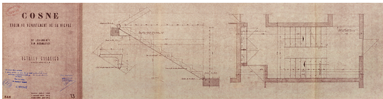
Opération de 32 logements, plans de détails des escaliers, L. Robert et M. Guillaume, avril 1955. (Archives municipales Cosne-Cours-sur-Loire, 200 W 16 - PC 722)
