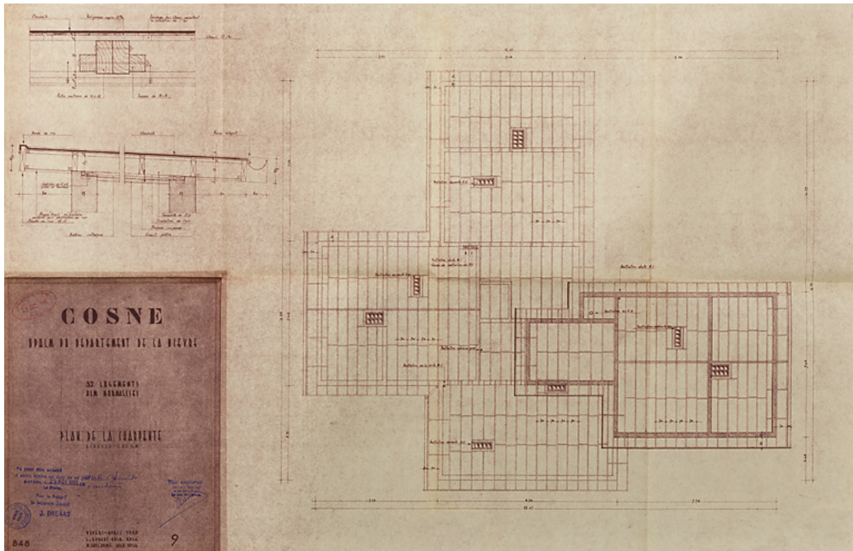
Opération de 32 logements, plan de la charpente, L. Robert et M. Guillaume, avril 1955. (Archives municipales Cosne-Cours-sur-Loire, 200 W 16 - PC 722)
