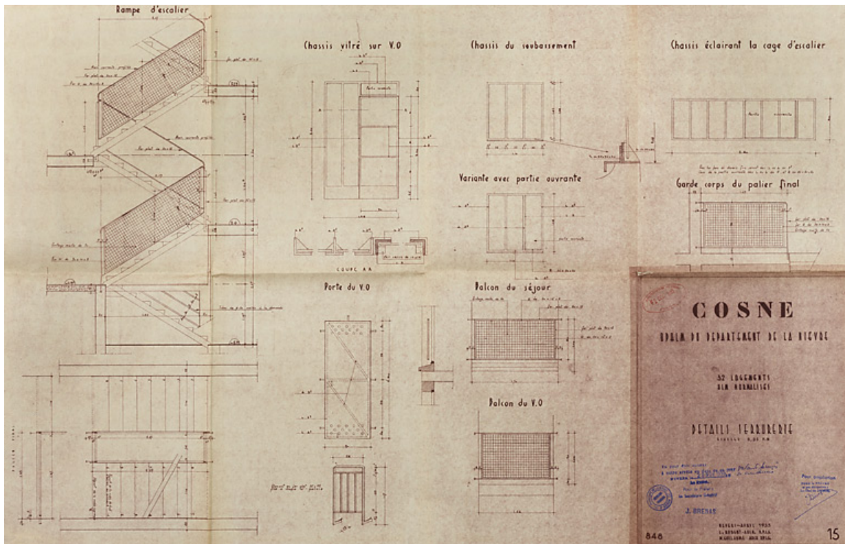
Opération de 32 logements, plans et élévations de détails de serrurerie, L. Robert et M. Guillaume, avril 1955. (Archives municipales Cosne-Cours-sur-Loire, 200 W 16 - PC 722) 58, Cosne-Cours-sur-Loire rue Fernand Petit
