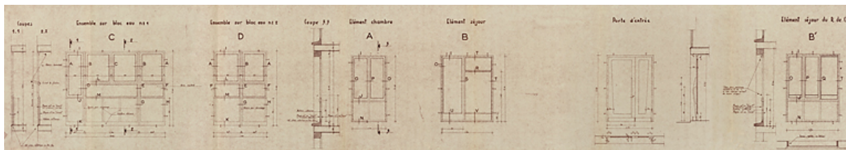
Opération de 32 logements, plans et élévations de détails des menuiseries, L. Robert et M. Guillaume, avril 1955. (Archives municipales Cosne-Cours-sur-Loire, 200 W 16 - PC 722)
