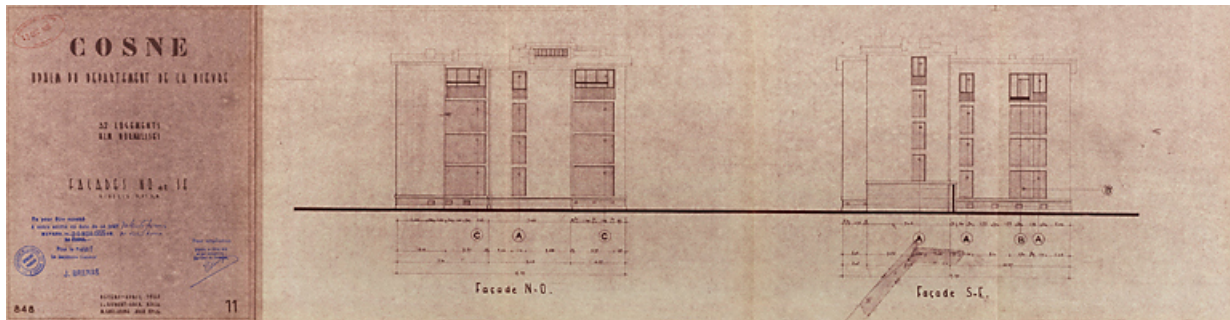
Opération de 32 logements, élévations des façades nord-ouest et sud-est, L. Robert et M. Guillaume, avril 1955. (Archives municipales Cosne-Cours-sur-Loire, 200 W 16 - PC 722)
