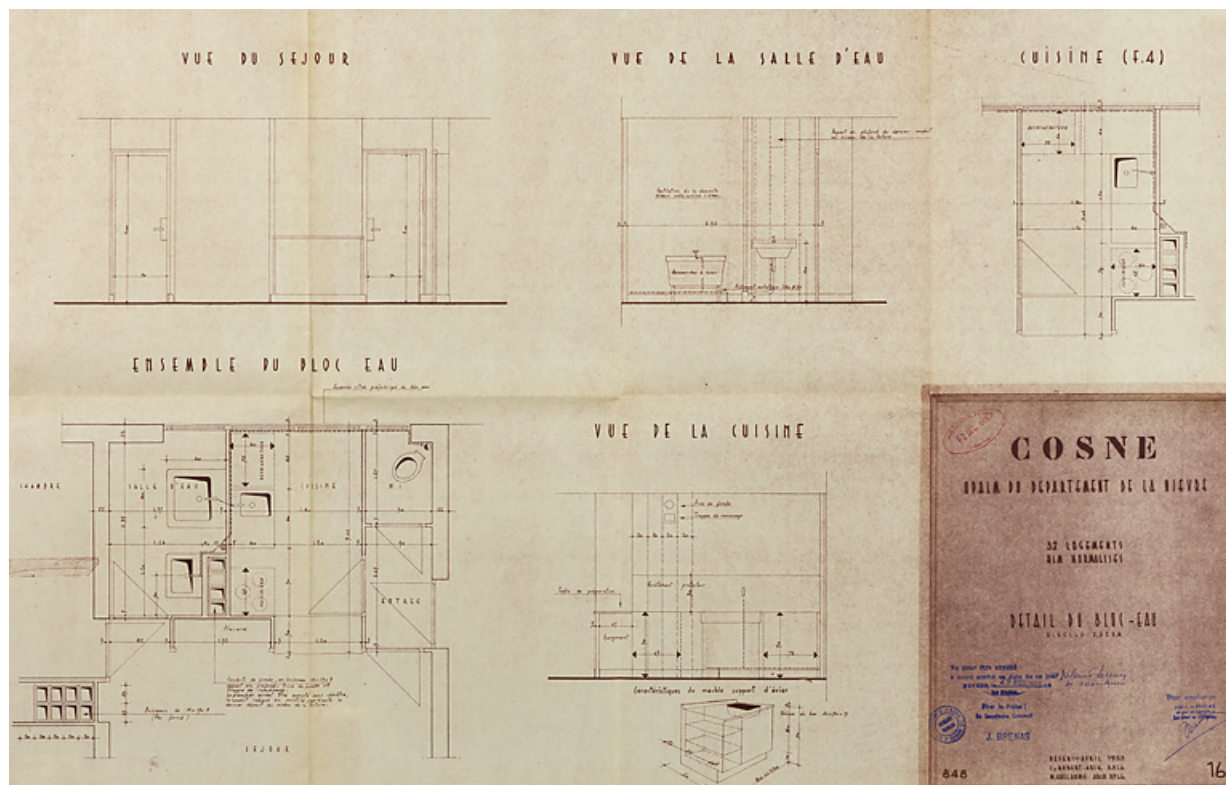
Opération de 32 logements, plans et élévations de détails du bloc-eau, L. Robert et M. Guillaume, avril 1955. (Archives municipales Cosne-Cours-sur-Loire, 200 W 16 - PC 722) 58, Cosne-Cours-sur-Loire rue Fernand Petit
