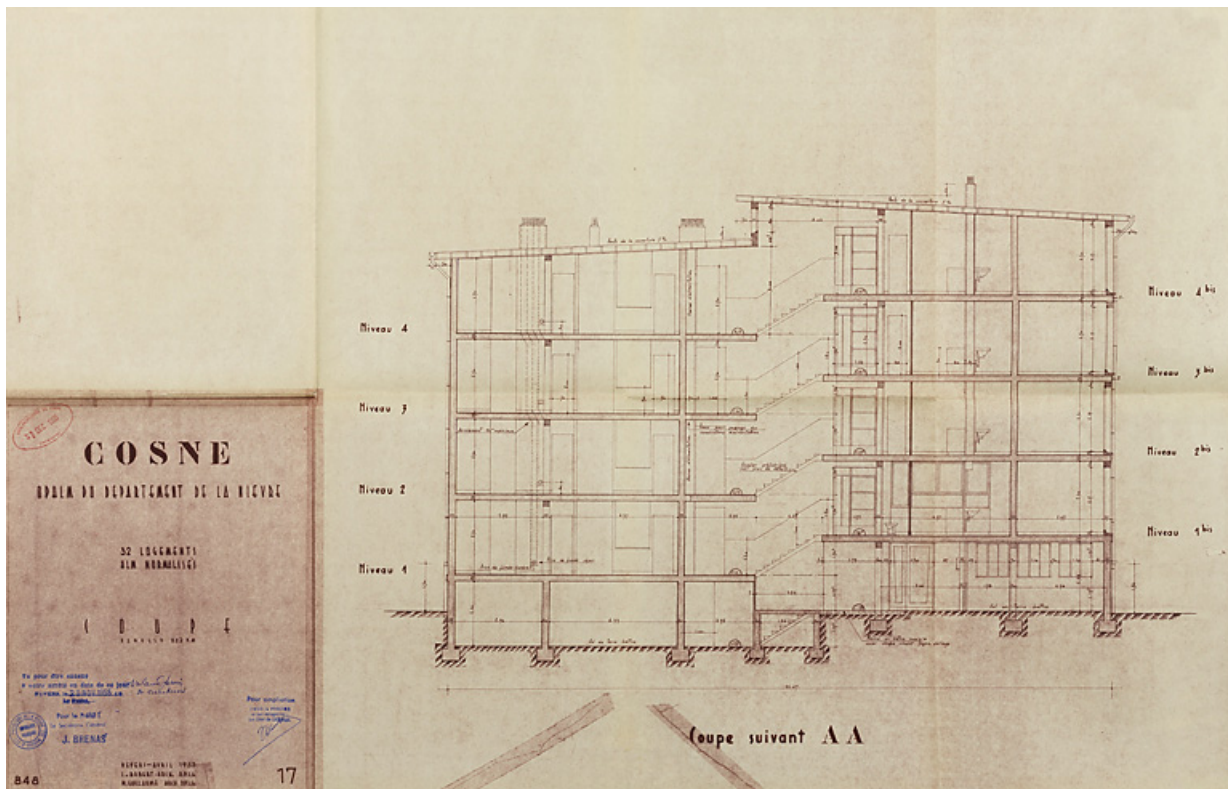
Opération de 32 logements, coupe, L. Robert et M. Guillaume, avril 1955. (Archives municipales Cosne-Cours-sur-Loire, 200 W 16 - PC 722)
