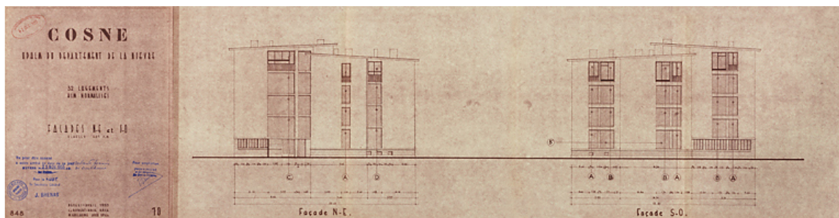
Opération de 32 logements, élévations des façades nord-est et sud-ouest, L. Robert et M. Guillaume, avril 1955. (Archives municipales Cosne-Cours-sur-Loire, 200 W 16 - PC 722)
