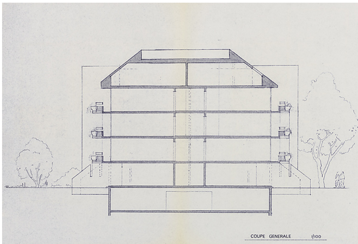
Opération de 132 logements : coupe générale des immeubles ; F. Martin Lavigne, D. Chenut, O. Senly, septembre 1979. (Archives municipales Cosne-Cours-sur-Loire, 200 W 115 - PC 684)
