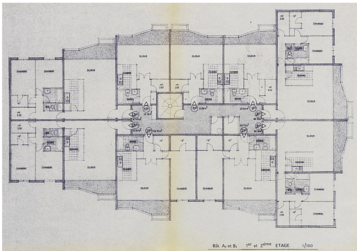
Opération de 132 logements : bâtiments A et B, plan du premier et du deuxième étages ; F. Martin Lavigne, D. Chenut, O. Senly, septembre 1979. (Archives municipales Cosne-Cours-sur-Loire, 200 W 115 - PC 684)
