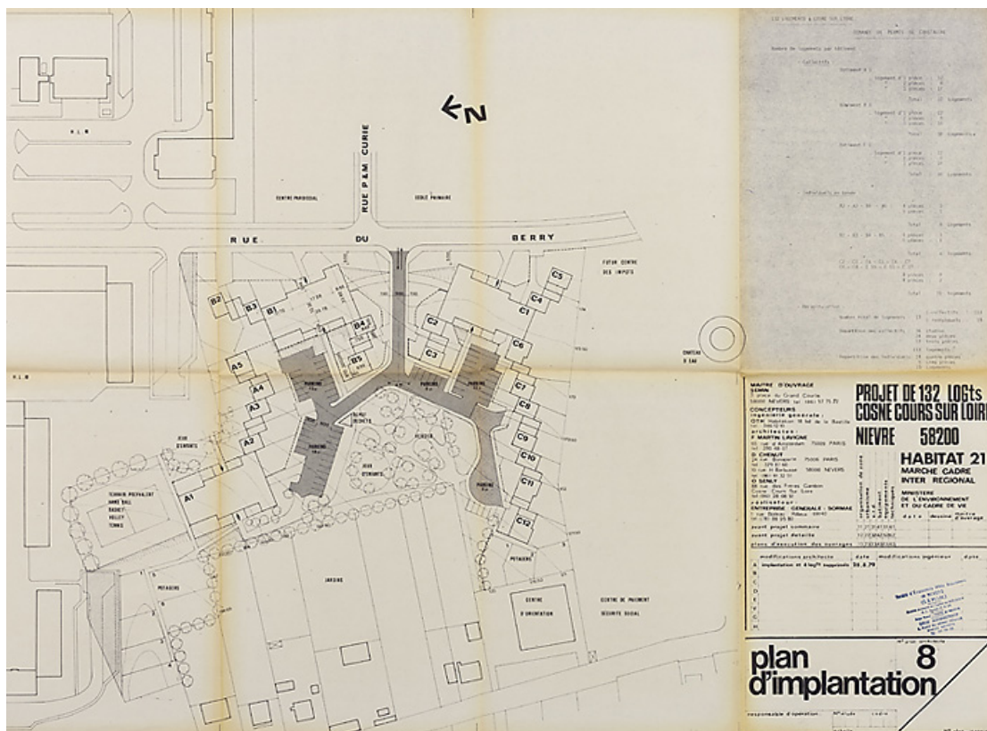
Opération de 132 logements : plan d'implantation ; F. Martin Lavigne, D. Chenut, O. Senly, août 1979. (Archives municipales Cosne-Cours-sur-Loire, 200 W 115 - PC 684)
