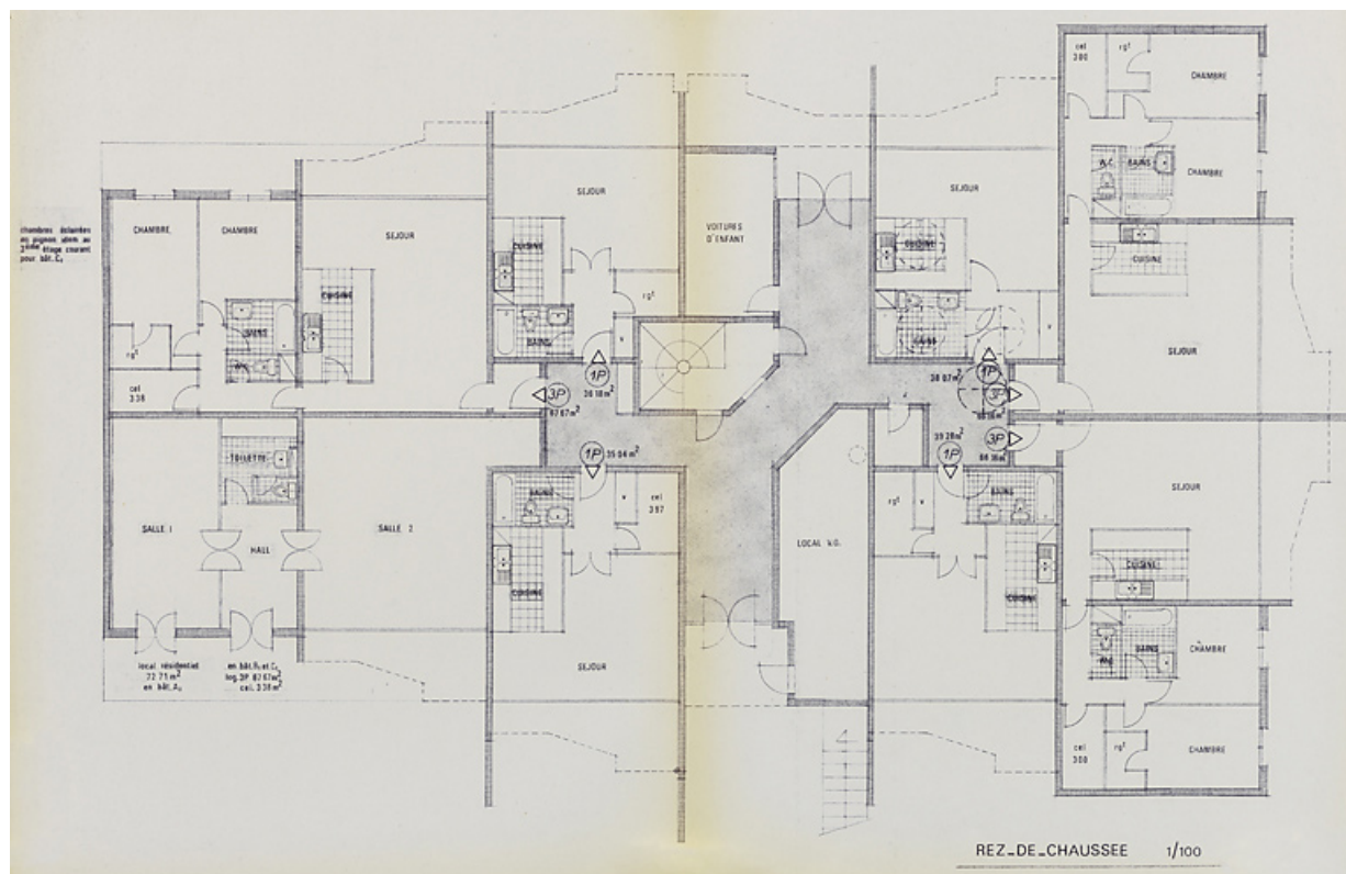
Opération de 132 logements : plan du rez-de-chaussée des immeubles ; F. Martin Lavigne, D. Chenut, O. Senly, septembre 1979. (Archives municipales Cosne-Cours-sur-Loire, 200 W 115 - PC 684) 58, Cosne-Cours-sur-Loire allée du Berry
