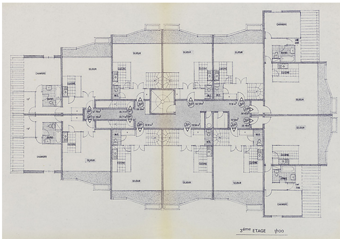
Opération de 132 logements : plan du troisième étage des immeubles ; F. Martin Lavigne, D. Chenut, O. Senly, septembre 1979. (Archives municipales Cosne-Cours-sur-Loire, 200 W 115 - PC 684)
