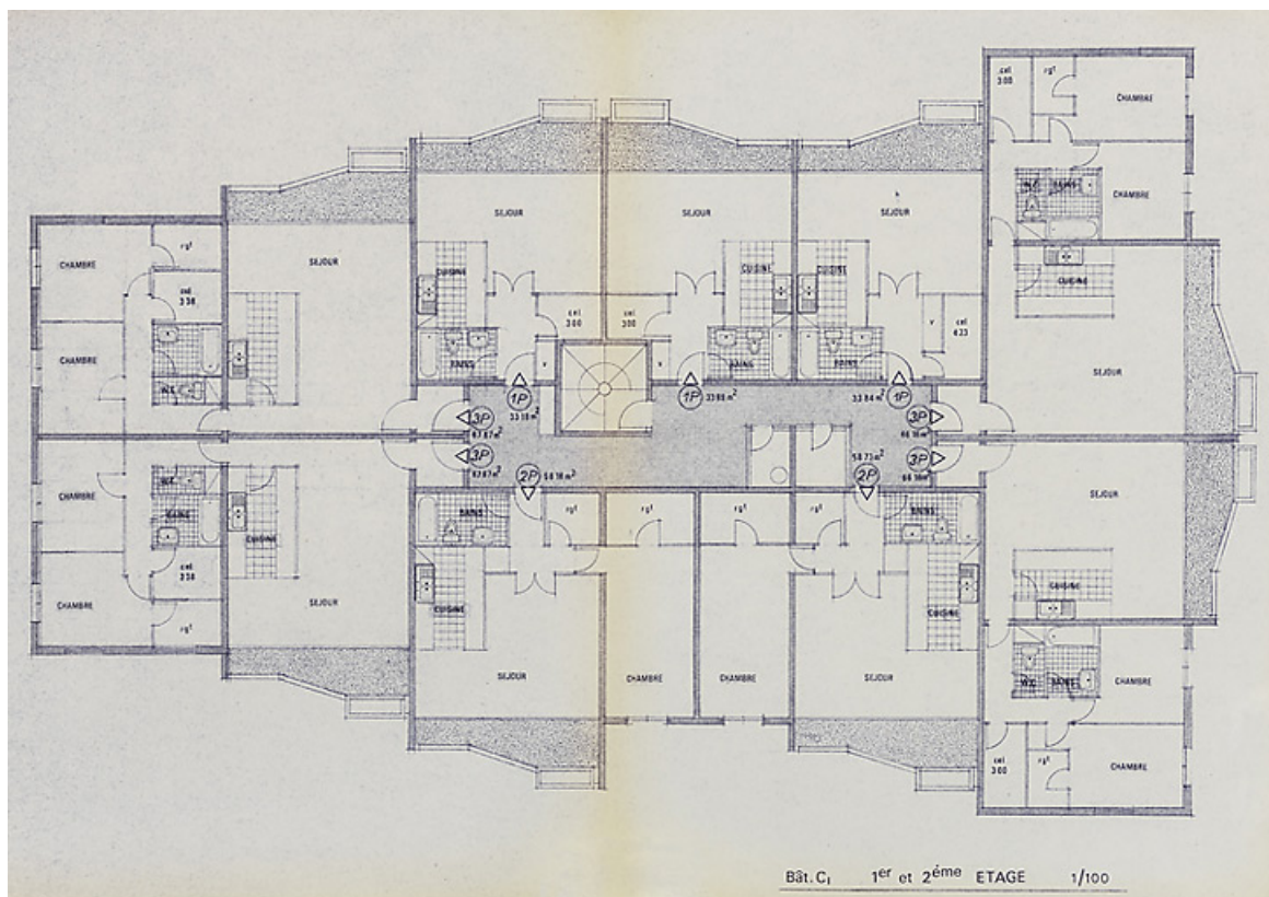
Opération de 132 logements : bâtiment C, plan du premier et du deuxième étages ; F. Martin Lavigne, D. Chenut, O. Senly, septembre 1979. (Archives municipales Cosne-Cours-sur-Loire, 200 W 115 - PC 684)
