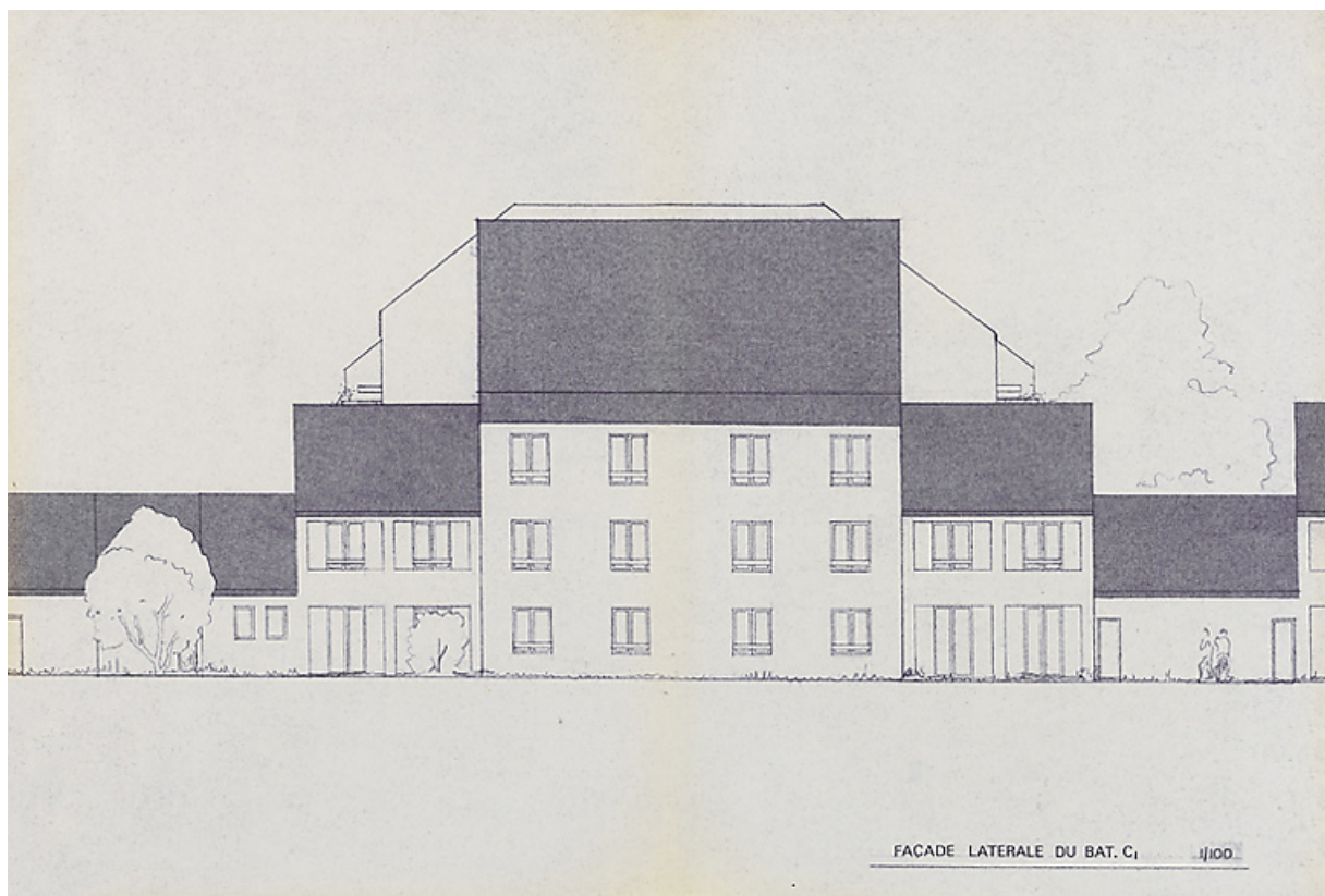
Opération de 132 logements : façade latérale du bâtiment C ; F. Martin Lavigne, D. Chenut, O. Senly, septembre 1979. (Archives municipales Cosne-Cours-sur-Loire, 200 W 115 - PC 684)
