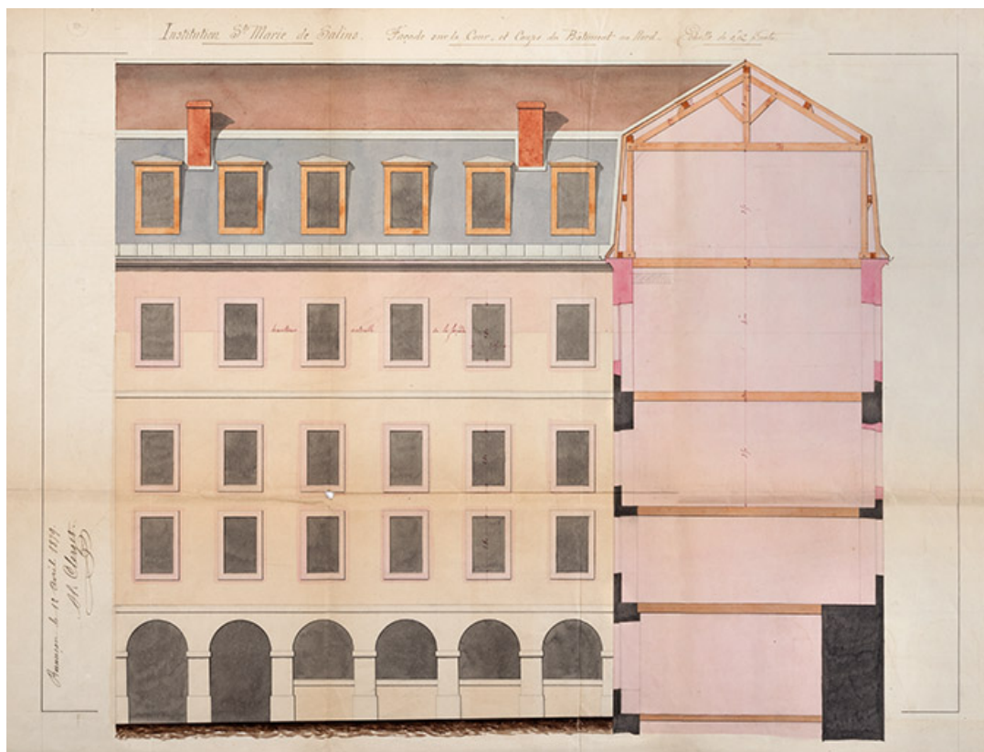
Institution Sainte-Marie de Salins. Façade sur la cour et coupe du bâtiment nord, 1879.
