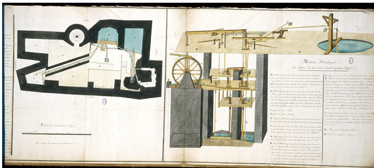
Plan des Sources du puit à Muire, a la petite Saline [et] Machines Hydrauliques Qui Elèvent Les Eaux salées et douces du puit à Muire.
