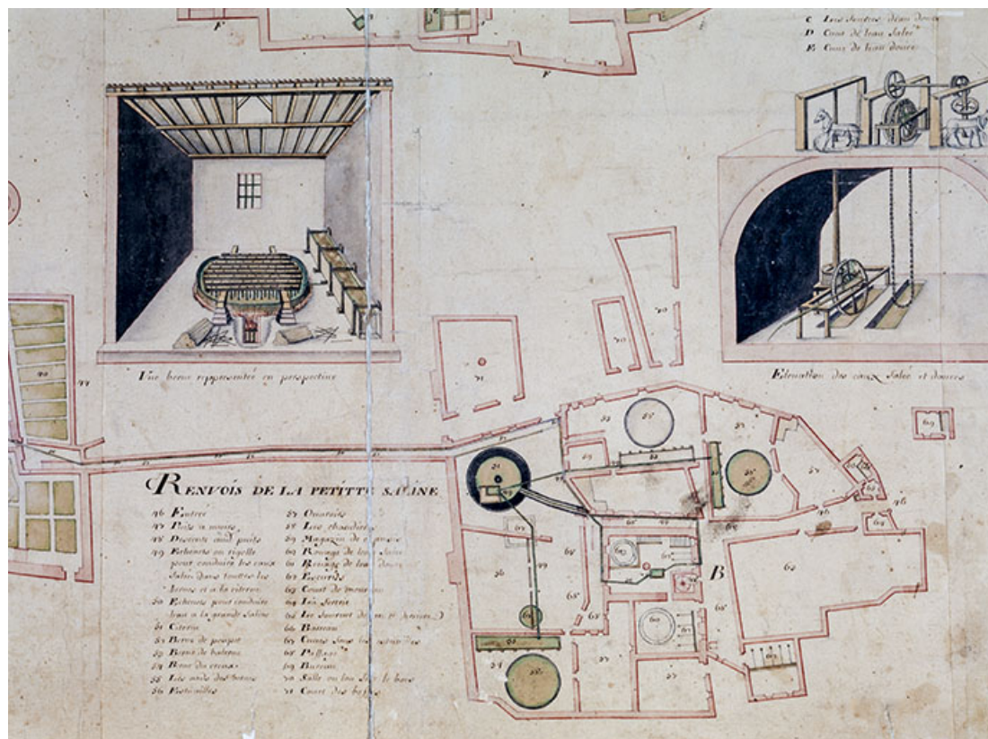
Plan géométral du Rets de chaussée [... : détail du rez-de-chaussée de la Petite Saline et des vues perspectives]. 39, Salins-les-Bains, 2 place des Alliés et de la Résistance
