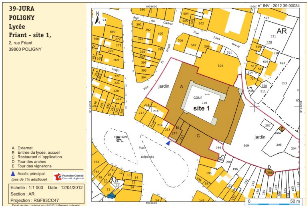
Plan-masse et de situation. Extrait du plan cadastral numérisé , 2012, section AR , échelle 1 / 1 000.
