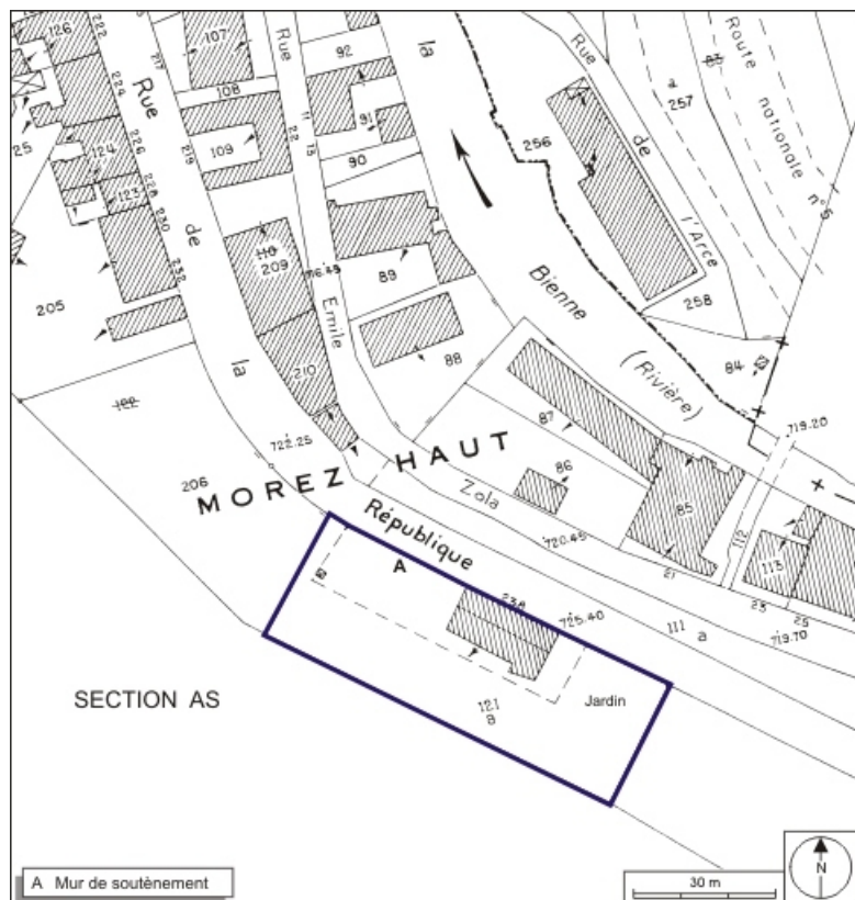
Plan-masse et de situation. Extrait du plan cadastral, 1980, section AK, échelle 1:1000. 39, Morez, 238 rue de la République
