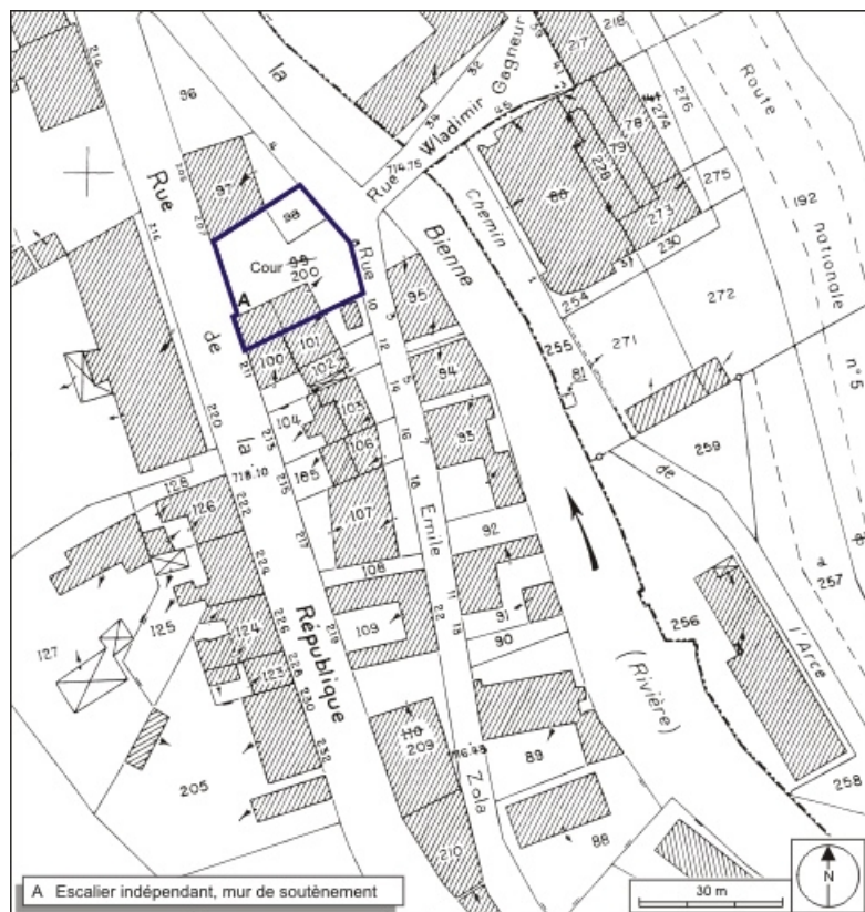
Plan-masse et de situation. Extrait du plan cadastral, 1980, section AK, échelle 1:1000. 39, Morez, 209 rue de la République
