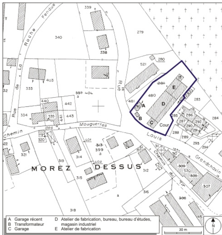
Plan-masse et de situation. Extrait du plan cadastral, 1980, section AI, échelle 1:1000. 39, Morez, 18 rue Louis Grandchavin
