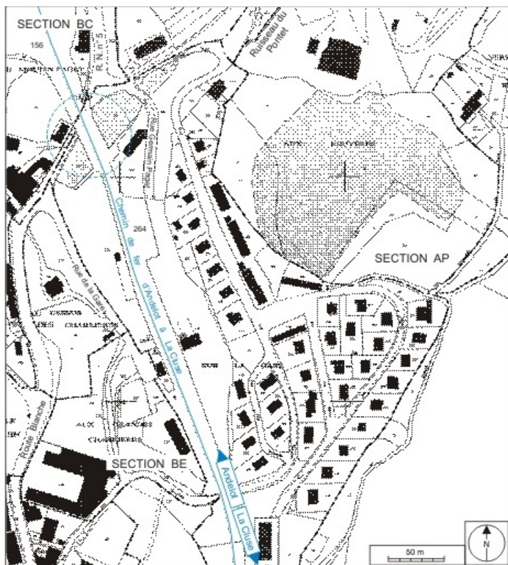
Plan-masse et de situation. Extrait du plan cadastral informatisé, 2006, sections BC et BE, échelle 1:2500. 39, Morbier route Blanche
