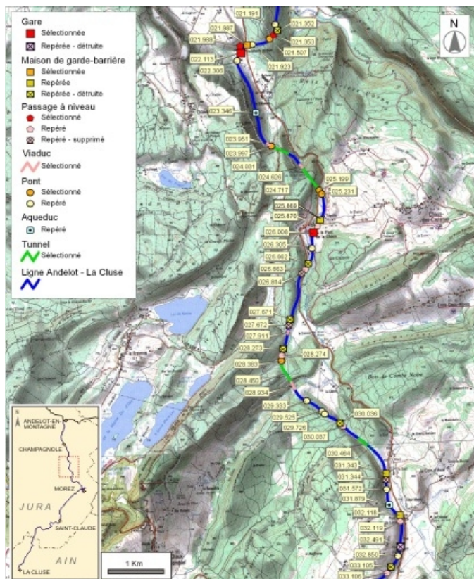
Carte et schéma de localisation des ouvrages : du Vaudieux à La Chaumusse. Carte topographique, IGN, 2000, dalles F087-048 et F087-049, échelle 1:48 000. Scan 25, licence n° 2008/CISE/2968.
