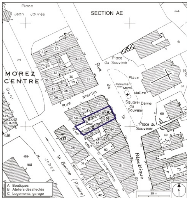
Plan-masse et de situation. Extrait du plan cadastral, 1980, section AI, échelle 1:1000. 39, Morez, 124, 126 rue de la République
