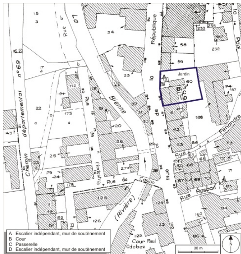
Plan-masse et de situation. Extrait du plan cadastral, 1980, section AE, échelle 1:1000. 39, Morez, 85 rue de la République
