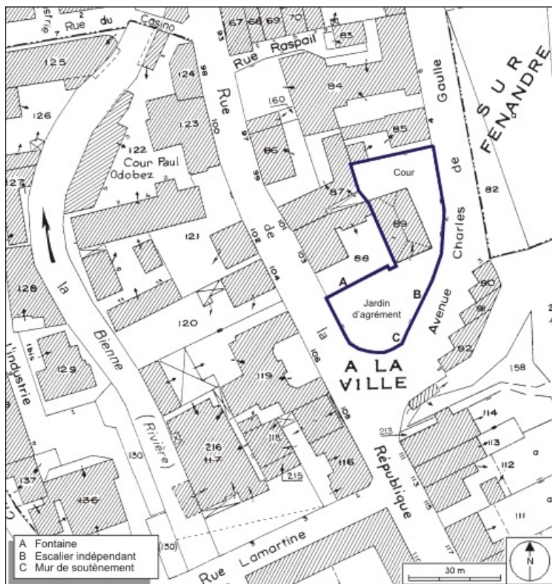
Plan-masse et de situation. Extrait du plan cadastral, 1980, section AE, échelle 1:1000. 39, Morez, 2 avenue Charles de Gaulle
