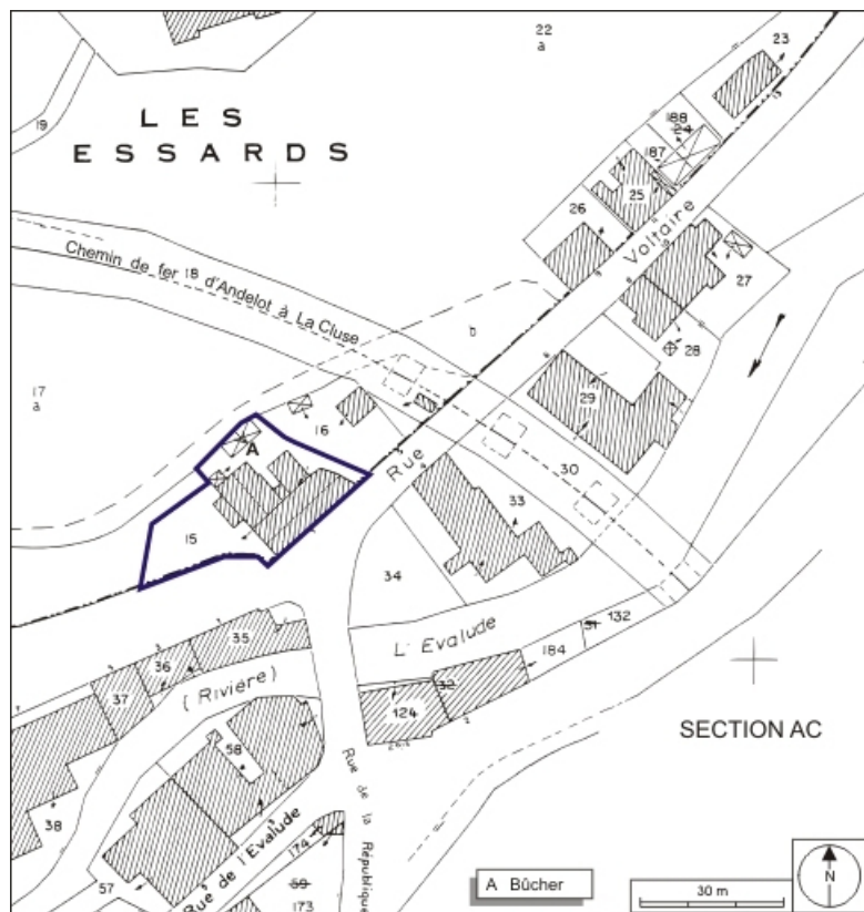
Plan-masse et de situation. Extrait du plan cadastral, 1980, section AB, échelle 1:1000. 39, Morez, 1 rue Voltaire
