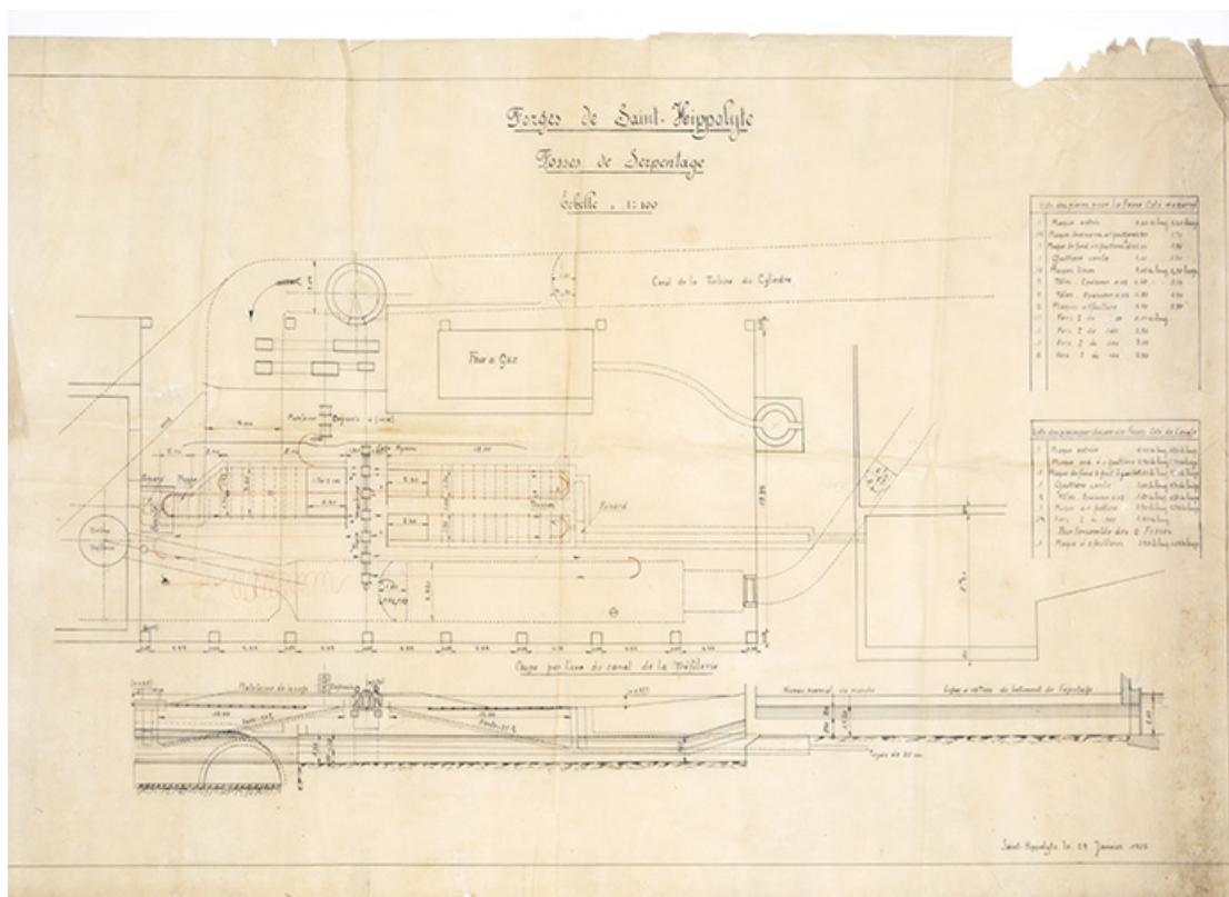
Forges de Saint-Hippolyte. Fosses de serpentage, 29 janvier 1925.
