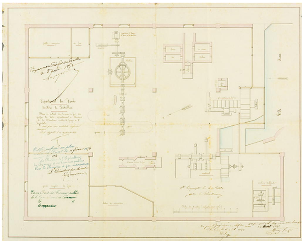
Plan de détail de l'usine à fer du Gouffre du Lod, appartenant à Monsieur A. de Blondeau, maître de forges à St Hippolyte, 14 septembre 1852.
