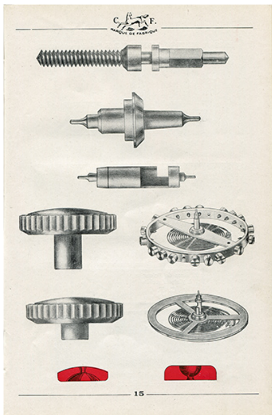
[Exemples de production de la société Cheval Frères : cylindre et axe, balancier-spiral, couronne de remontoir et rubis], 1950. 25, Maîche, 4 rue de la Gare
