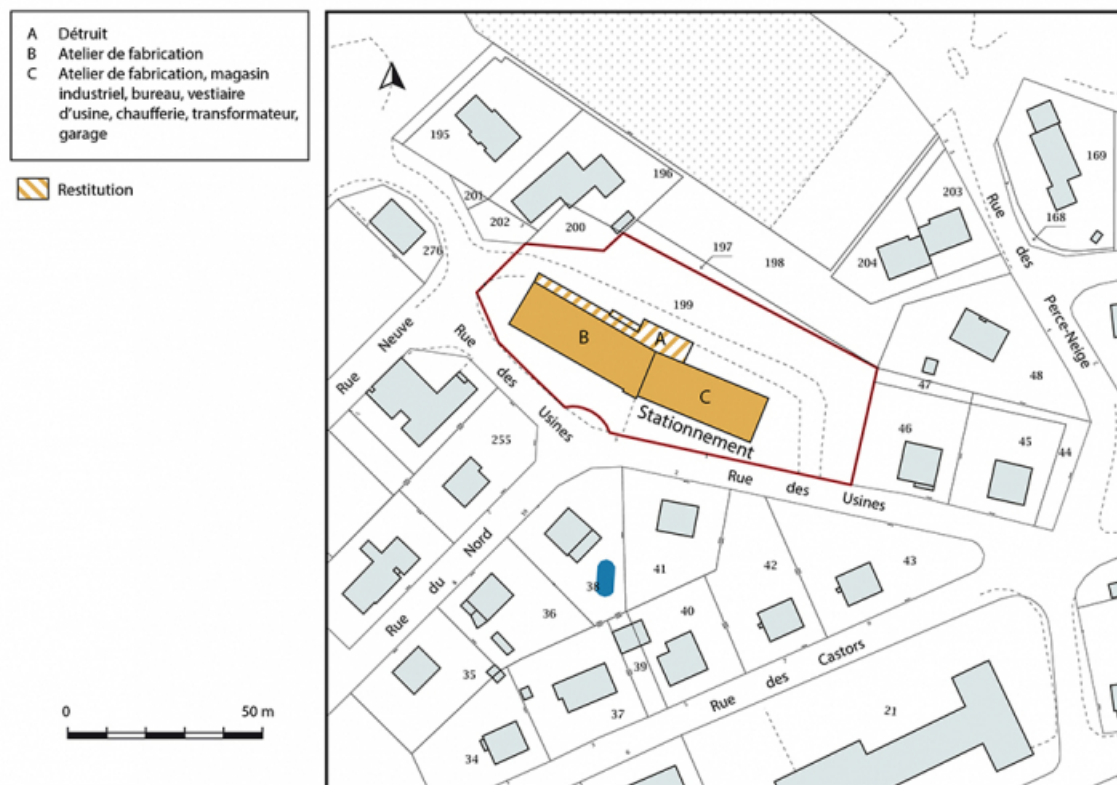
Plan-masse et de situation. Extrait du plan cadastral, 2018, section AO. 25, Le Russey, 1 et 5 rue des Usines
