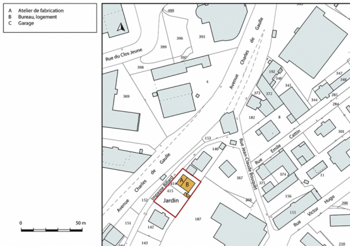
Plan-masse et de situation. Extrait du plan cadastral, 2018, section AF, 1/1 000. 25, Morteau, 14 impasse Billard
