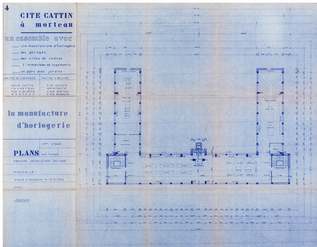
Cité Cattin à Morteau [...]. 4. La manufacture d'horlogerie. Plans 2ème étage. Ebauche, décolletage, taillage, 10 juin 1960. 25, Morteau, 8 avenue Charles de Gaulle
