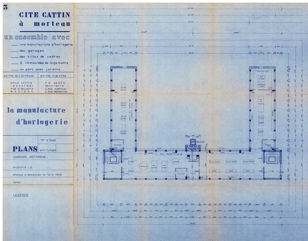
Cité Cattin à Morteau [...]. 3. La manufacture d'horlogerie. Plans 1er étage. Cadrons, nettoyage, 10 juin 1960. 25, Morteau, 8 avenue Charles de Gaulle
