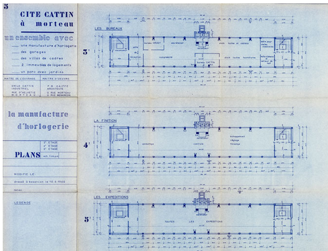
Cité Cattin à Morteau [...] 5. La manufacture d'horlogerie. Plans 3e étage [bureaux], 4e étage [finition], 5e étage [expédition], 10 juin 1960.
