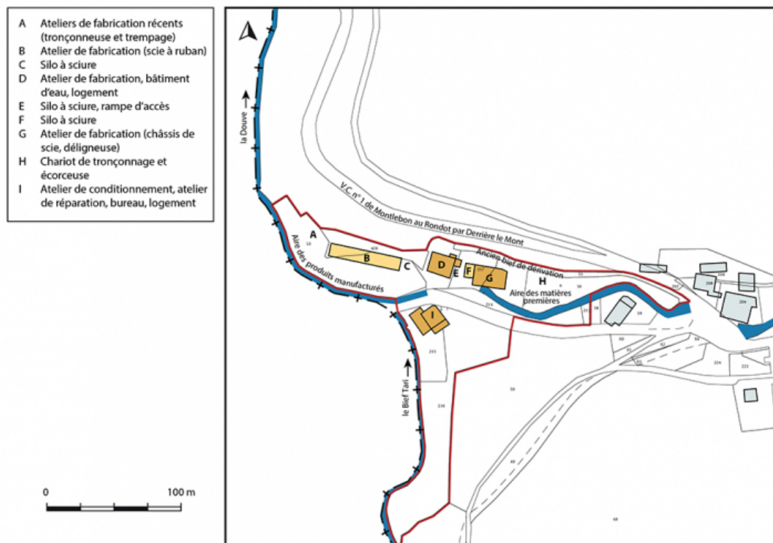
Plan-masse et de situation. Extrait du plan cadastral, 2016, section E, 1/2 500 agrandi à 1/2 000. 25, Montlebon, lieudit : Louadey
