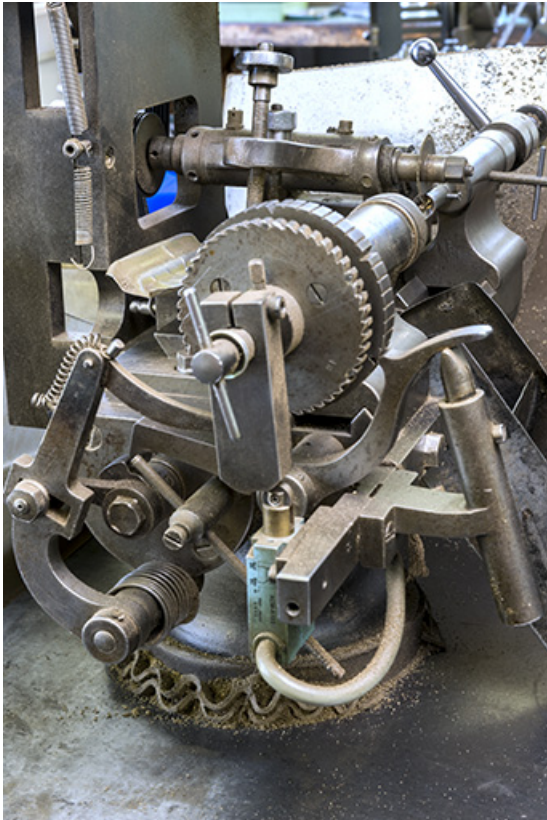
Machine à refendre les morilles : détail du système de commande (avec la fraise à refendre au second plan).
