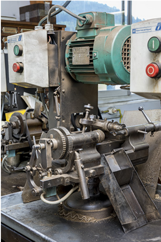
Machine à refendre les morilles (têtes de mandrin).
