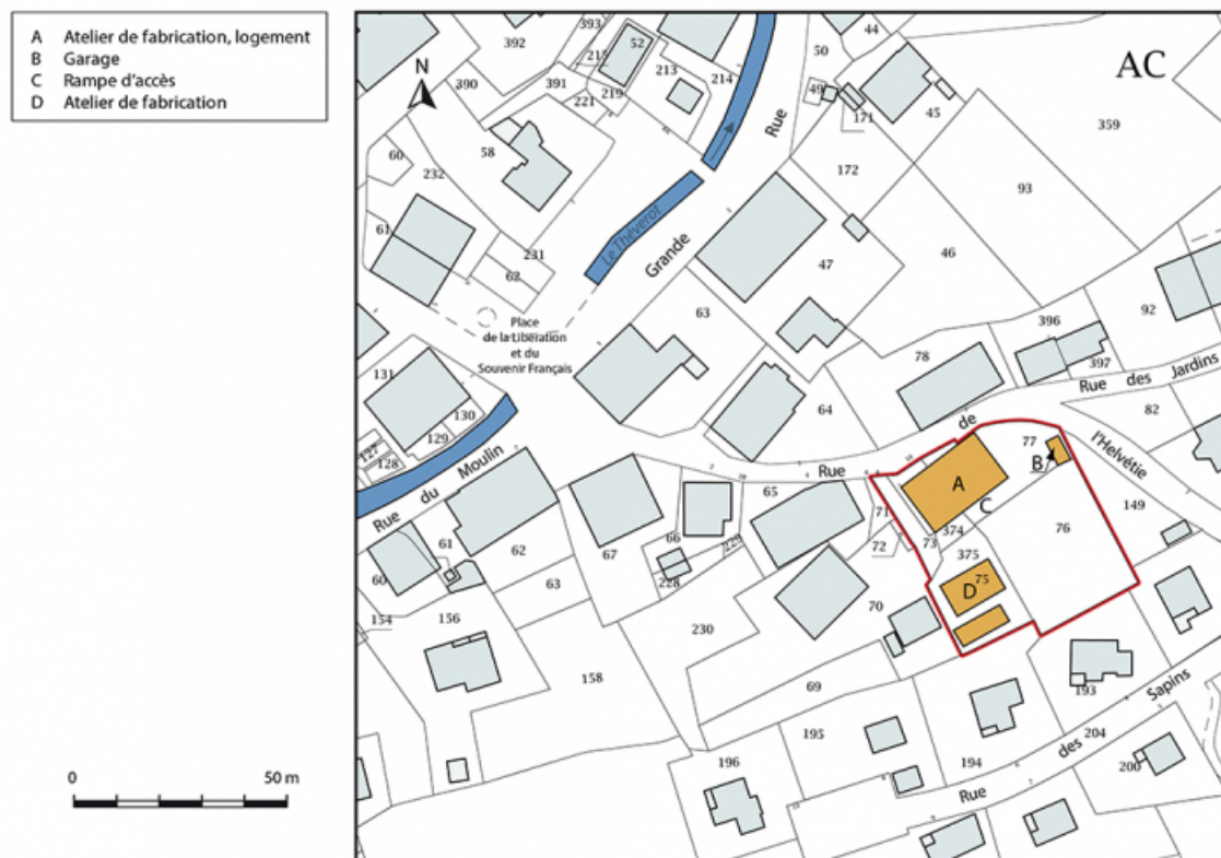
Plan-masse et de situation. Extrait du plan cadastral, 2017, section AC, 1/1 000. 25, Les Gras, 8-10 rue de l' Helvétie
