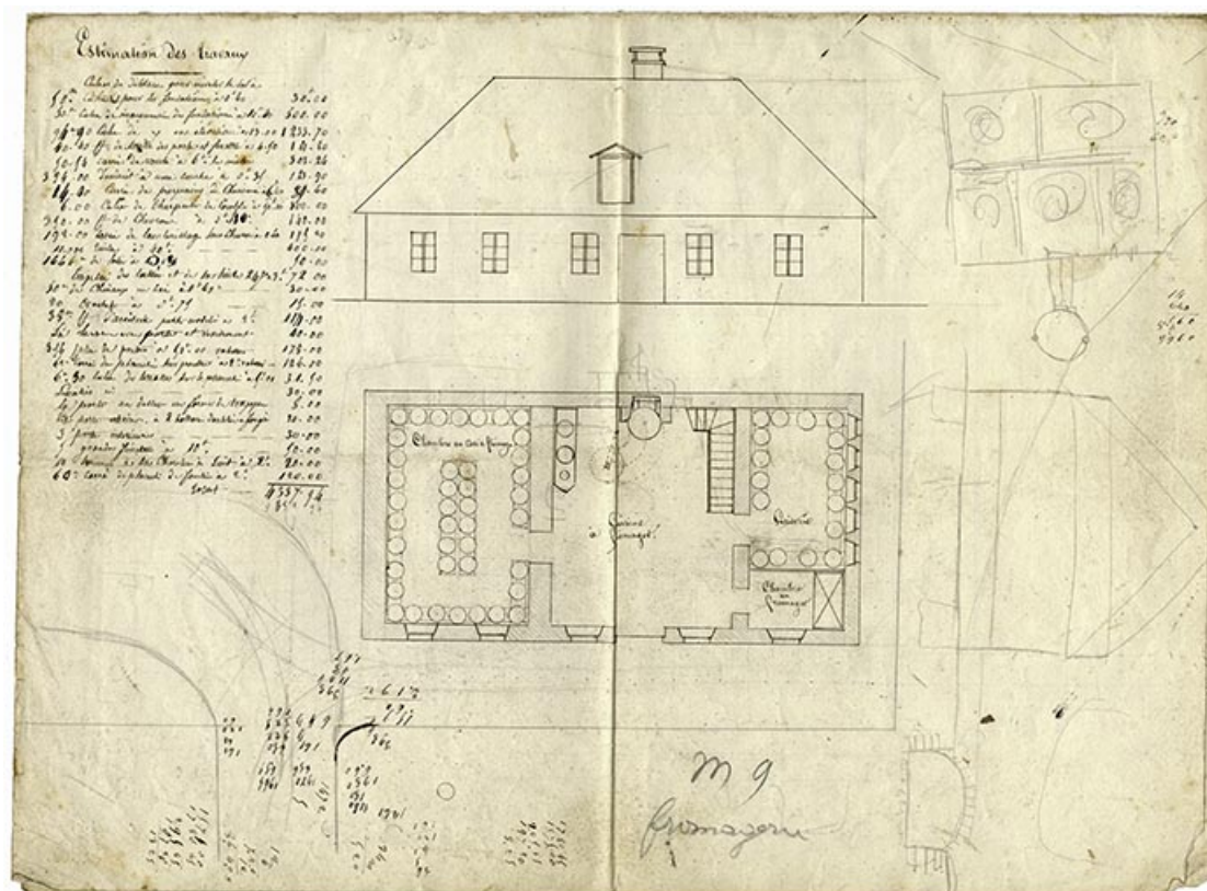
[Projet de fromagerie : plan et élévation], 1859.
