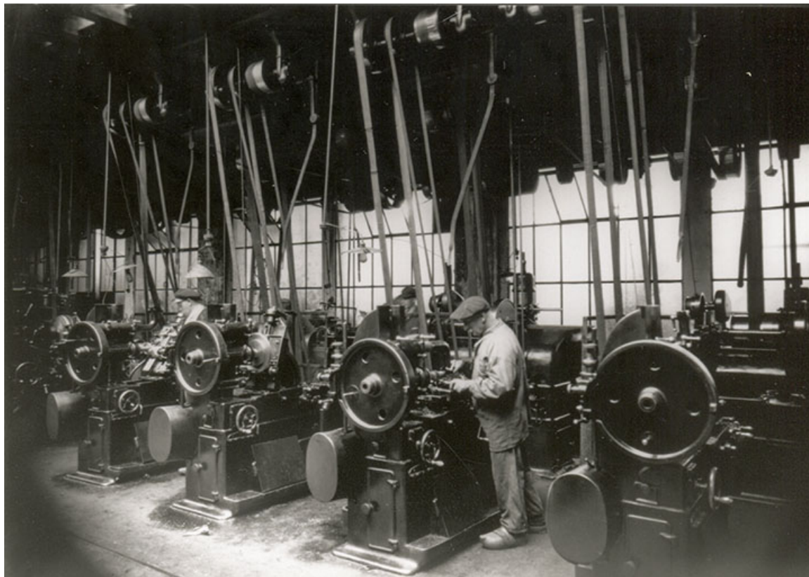
Machines-outils, phot. Stainacre, s.d. [début 20e siècle].
