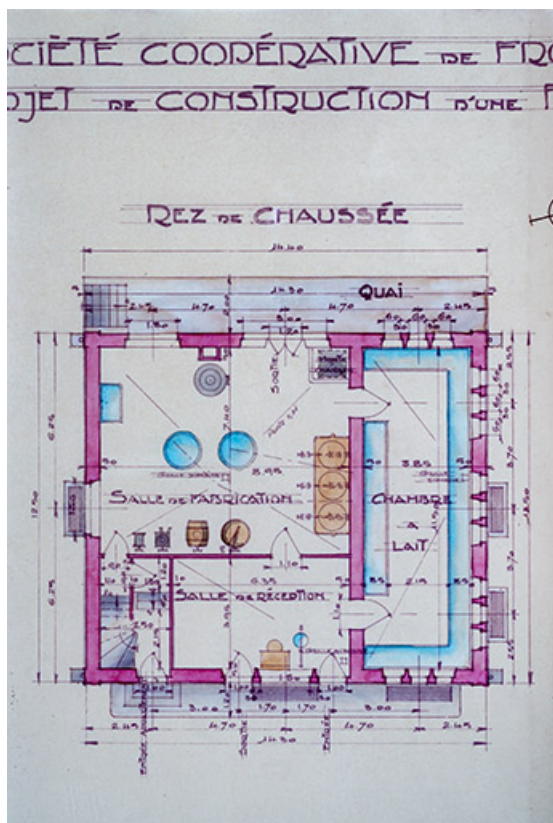
Société coopérative de fromagerie. Avant-projet de construction d'une fruitière - Plan du rez-de-chaussée, 1929. 25, Goux-les-Usiers, 23 rue des Ecoles
