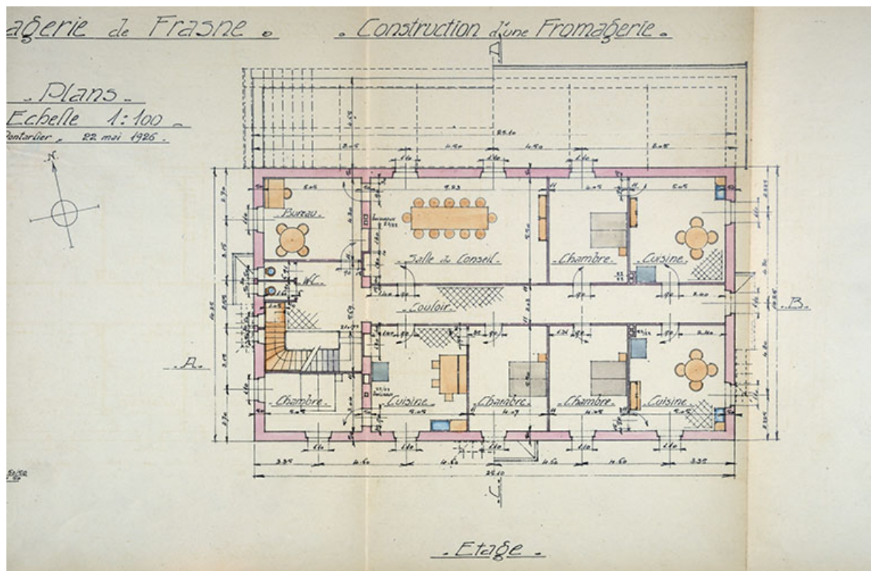
Société coopérative de fromagerie de Frasne. Construction d'une fromagerie, étage, 1926.
