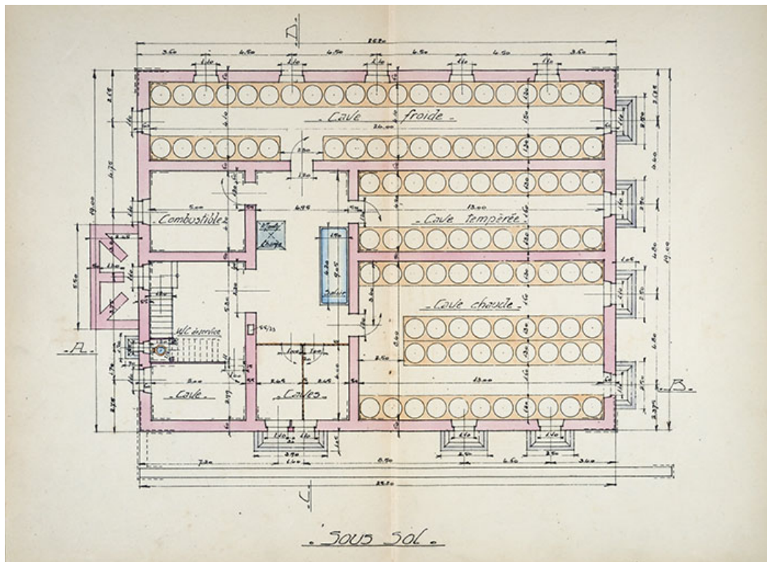
Société coopérative de fromagerie de Frasne. Construction d'une fromagerie, sous-sol, 1926. 25, Frasne, 2 rue de Bellevue
