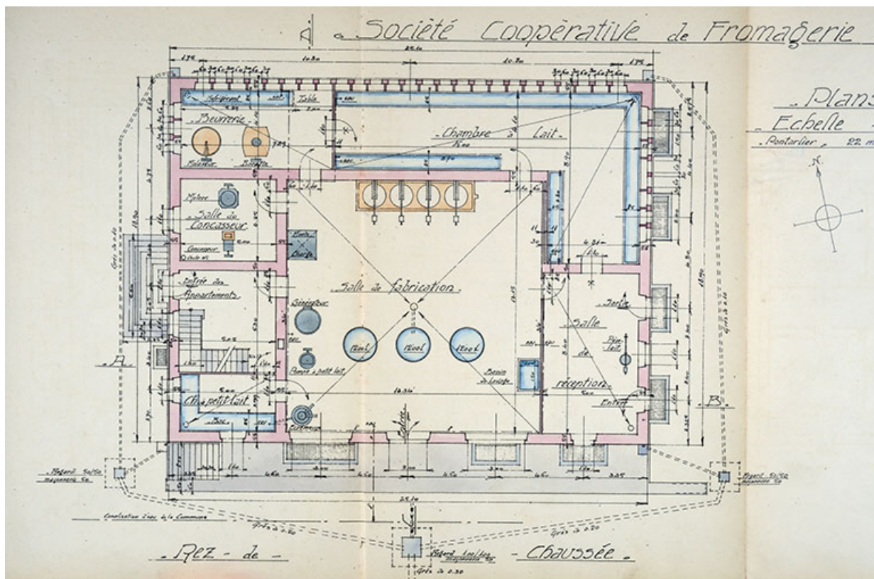
Société coopérative de fromagerie de Frasne. Construction d'une fromagerie, rez-de-chaussée, 1926. 25, Frasne, 2 rue de Bellevue
