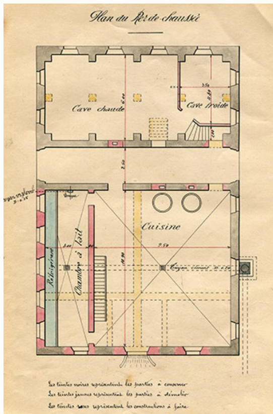
Transformation et réfection du chalet. Plan du rez-de-chaussée, 1902. 25, Courvières, 1 rue de Cuvier
