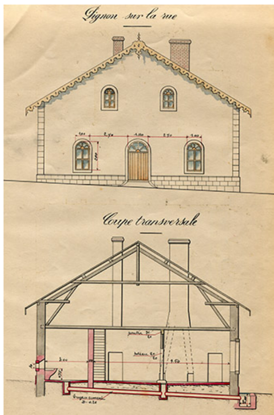
Transformation et réfection du chalet. Pignon sur rue et coupe transversale, 1902.
