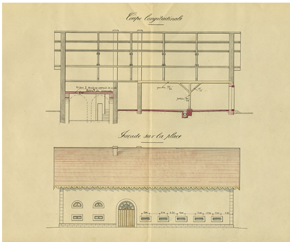
Transformation et réfection du chalet. Coupe longitudinale et façade sur la place, 1902.
