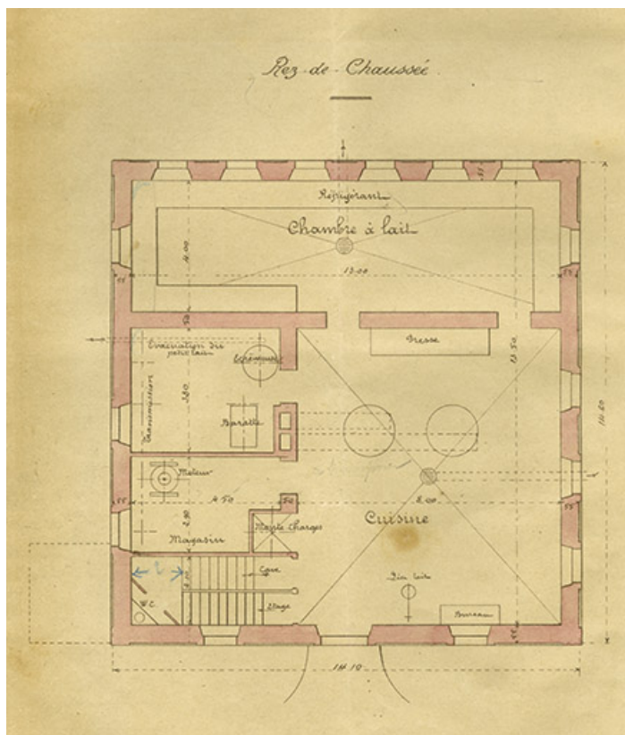
Construction d'un chalet-modèle. Plan du rez-de-chaussée, 1905.
