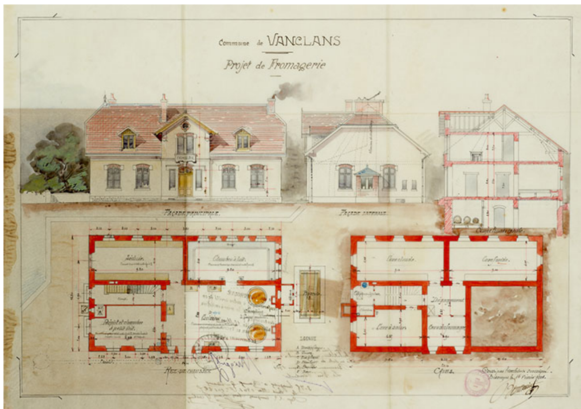
Commune de Vancians. Projet de fromagerie [façades, coupe et plans], 1901.
