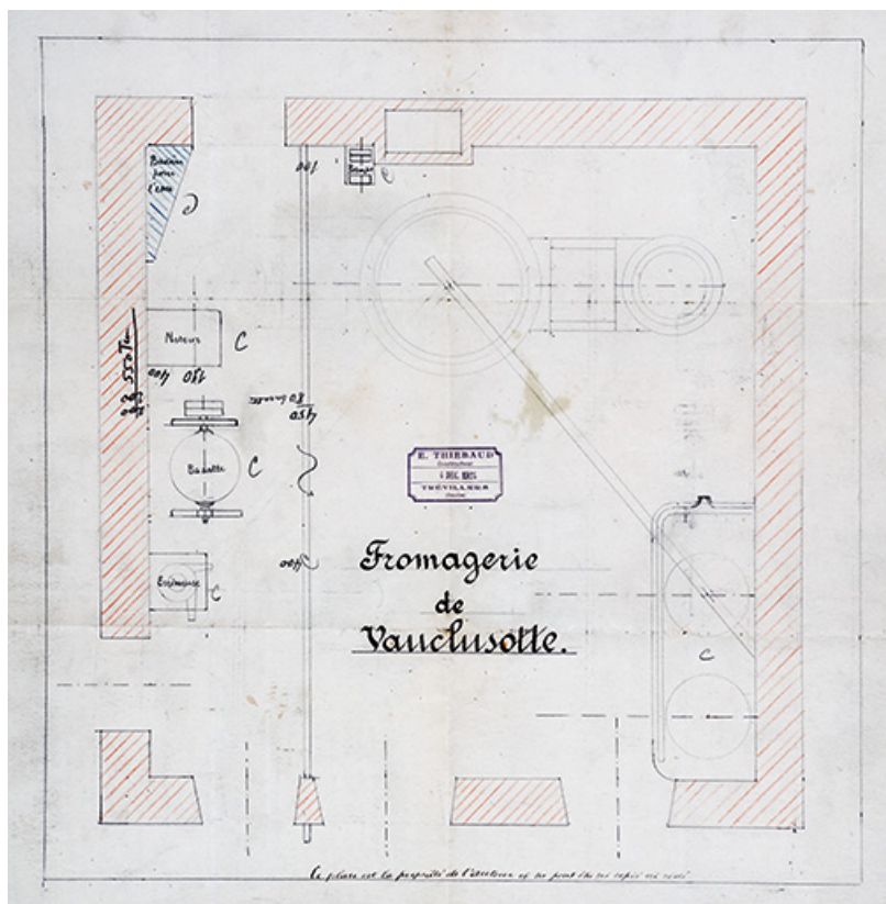
Fromagerie de Vaclusotte [schéma d'implantation de l'équipement], 1924. 25, Vaclusotte, 2 rue de la Fromagerie
