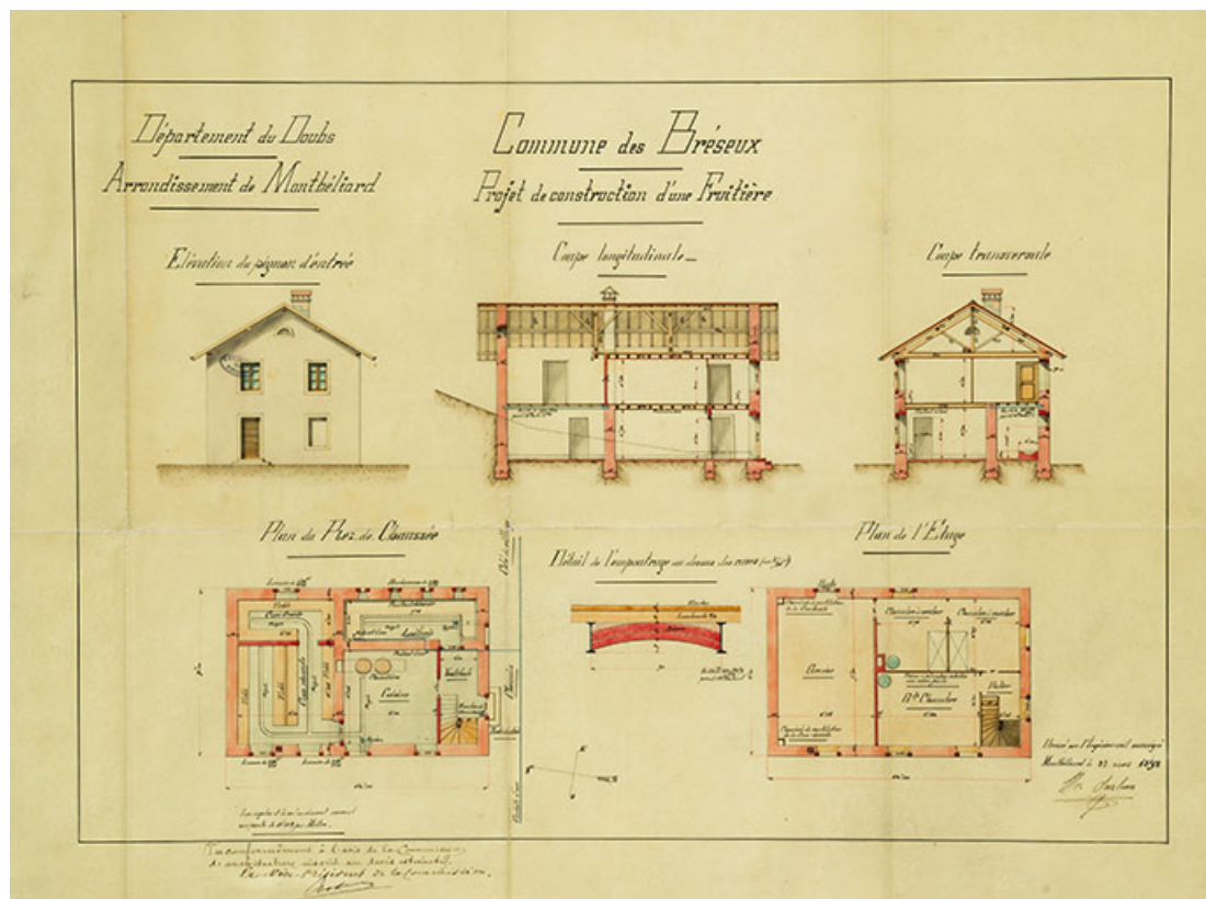
Commune des Bréseux. Projet de construction d'une fromagerie, 1892.
