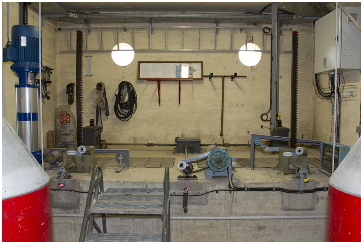
Barrage : commande des vannes de garde.
