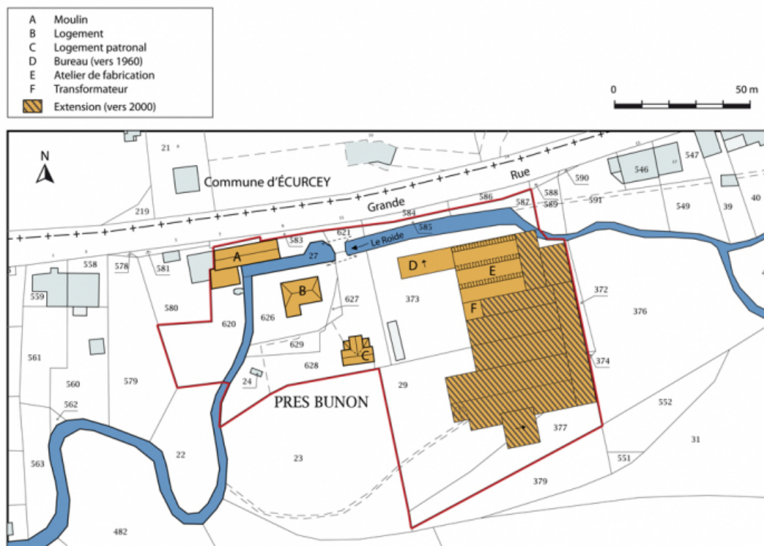
Plan-masse et de situation. Extrait du plan cadastral, 2015, section C. 25, Autechaux-Roide, 13 Grande-Rue
