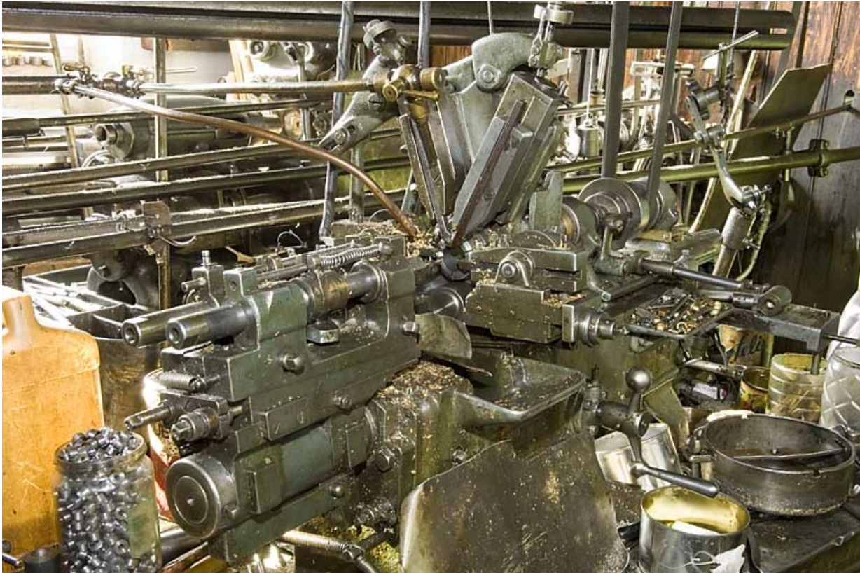
Détail d'un tour à décolleter Petermann (M). 25, Besançon, 11 rue Larmet
